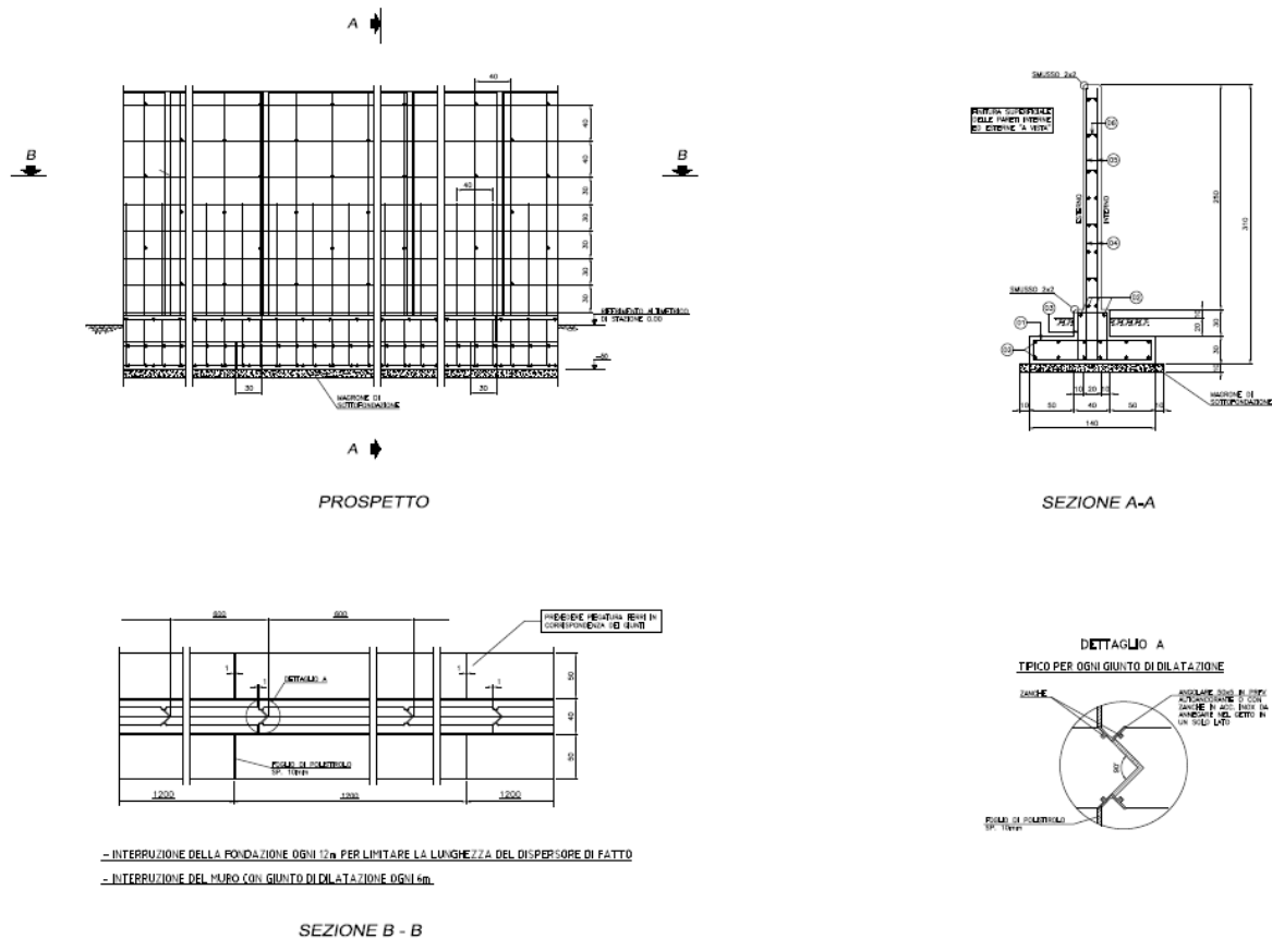
Figura 12 Recinzione stazione elettrica
