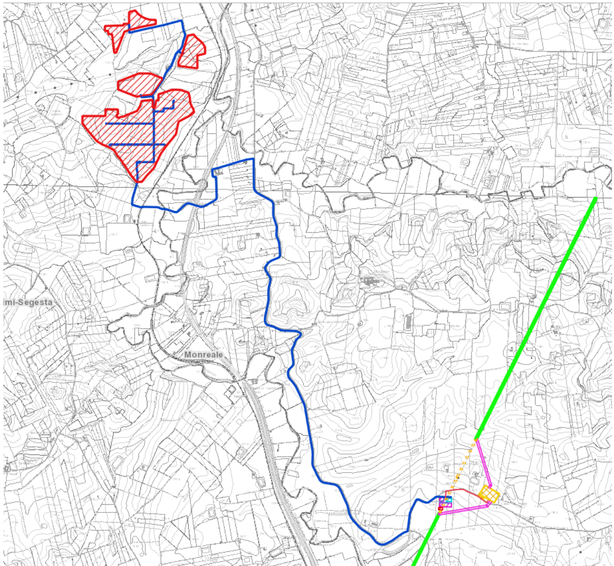
Figura 4 Area impianto fotovoltaico, cavidotto MT e area stazioni elettriche su IGM (elaborazione interna)
