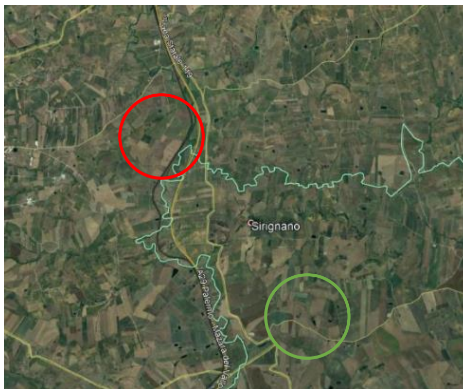
Figura 3 inquadramento geografico sito d'interesse su foto satellitare (impianto in rosso, stazioni elettriche in verde) (fonte Google LLC, elaborazione interna)
