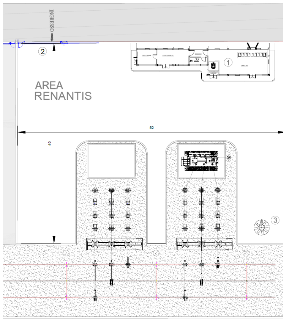
Figura 1 - Planimetria elettromeccanica della Stazione Trasformazione "Renantis Sicilia S.r.l."
