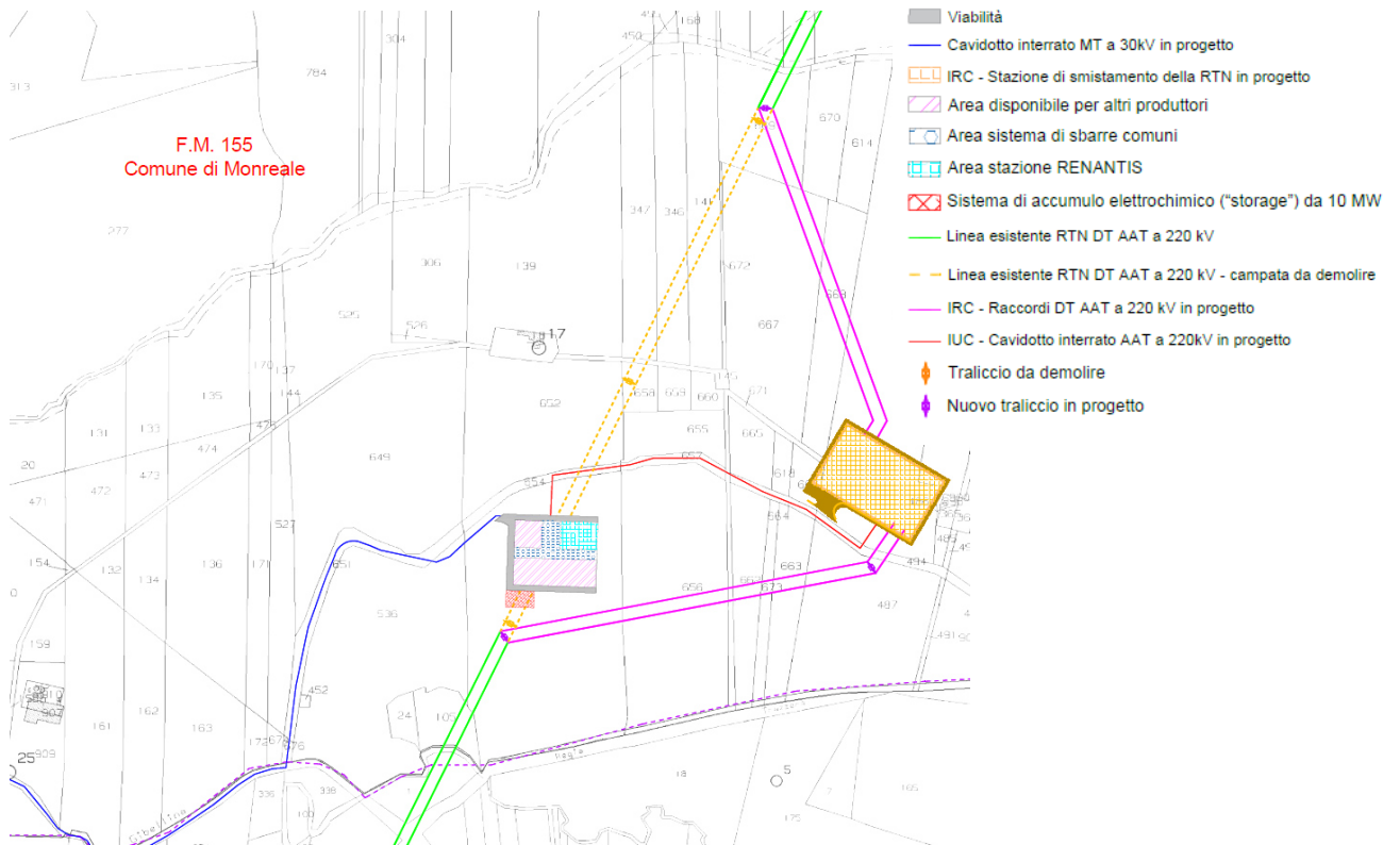
Figura 1.3.1 Stazioni elettriche per il collegamento alla Rete di Trasmissione Nazionale (RTN) su base catastale
