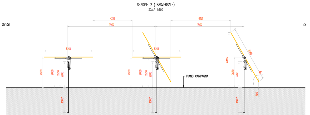
Particolare strutture sostegno moduli pannelli e distanze di campo (interfila m 9,5)
