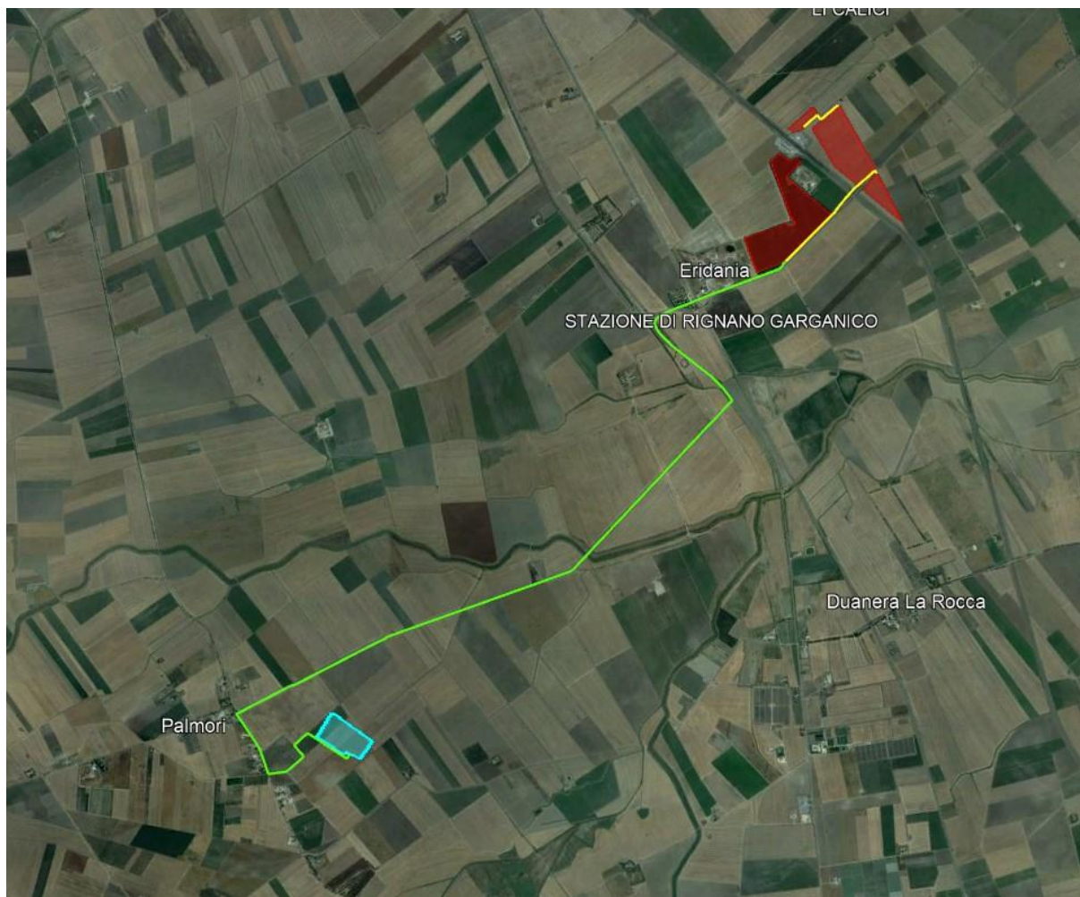
Figura 3.1: Soluzione di Connessione alla SE - In verde il percorso di connessione dal campo FV (aree rosse) al futuro ampliamento della SE (area azzurro)
