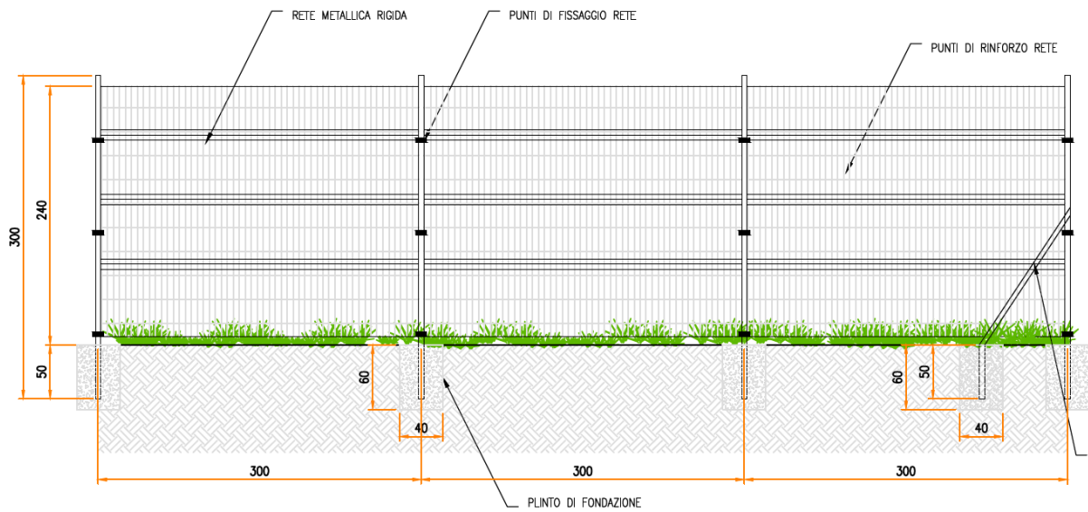
Figura 5.1: Particolare recinzione.
