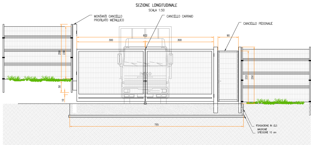
Figura 5.2: Particolare accesso.
