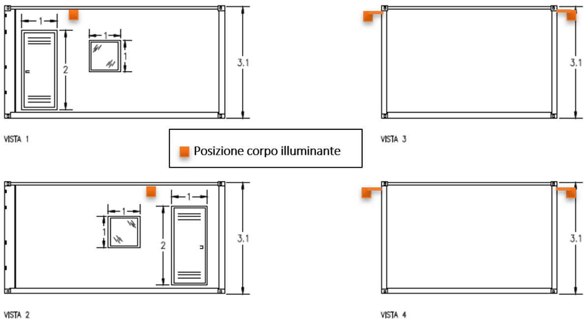
Figura 3.3: Tipologico Cabinato ufficio
