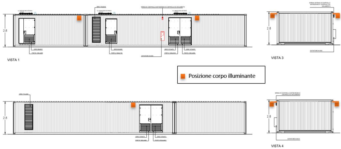
Figura 3.2: Tipologico Cabina di connessione con indicazione della posizione dei corpi illuminanti
