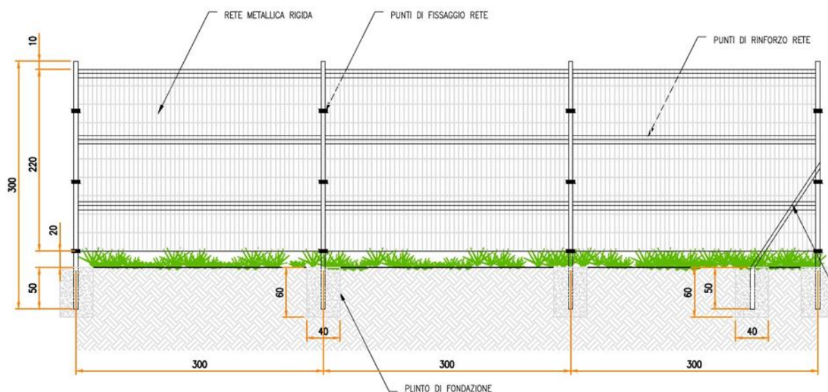
Figura 4.4: Particolare recinzione
