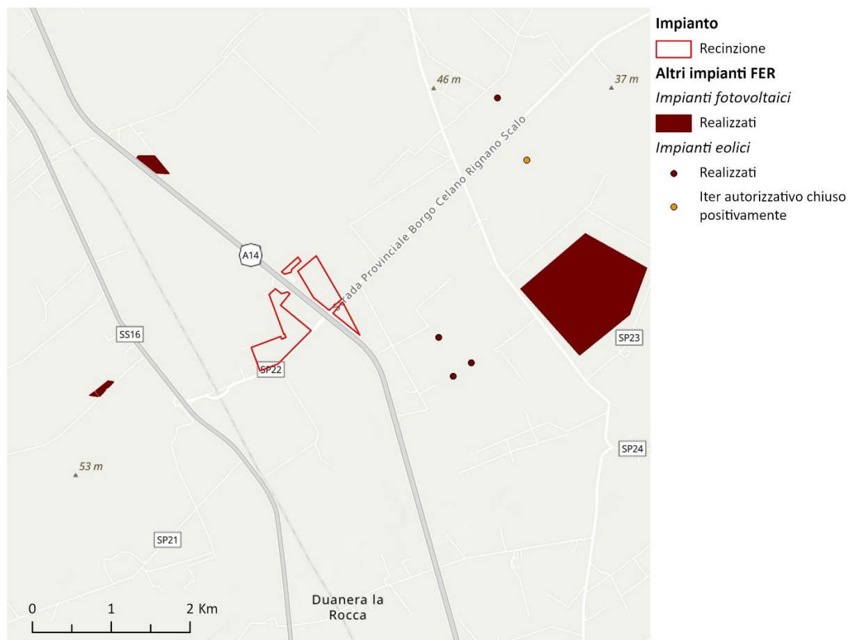
Figura 11.1: Impianto in progetto e altri impianti eolici/fotovoltaici presenti nell'area oggetto di studio – Elaborazione Montana S.p.A.
