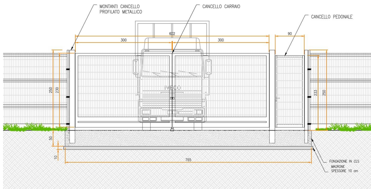
Figura 4.5: Particolare accesso
