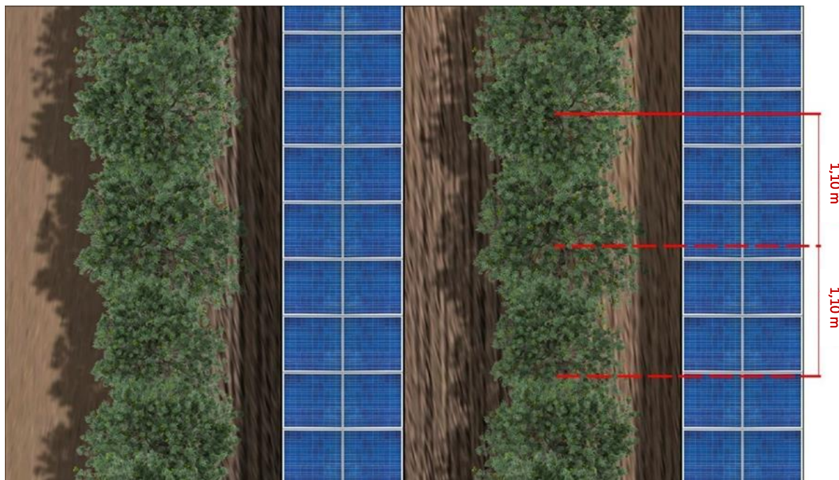
Figura 6.2: Tipologico - vista planimetrica dell'impianto olivicolo
