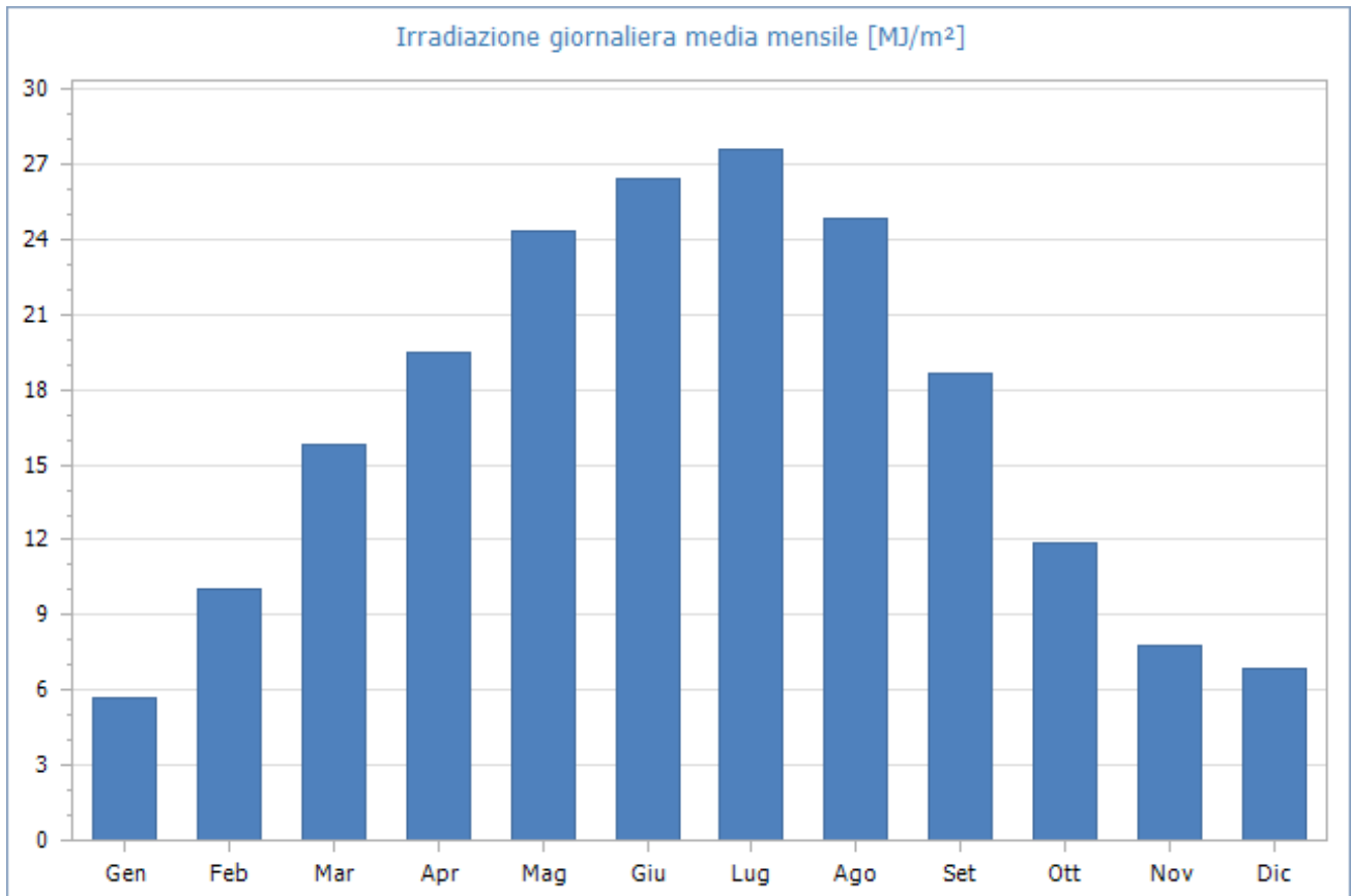
Fig. 2: Irradiazione giornaliera media mensile sul piano orizzontale [MJ/m²]- Fonte dati: Photovoltaic Geographical Information System (PVGIS)
