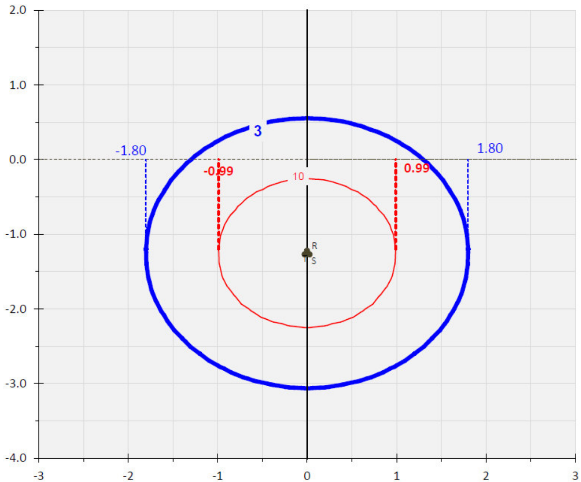
Curve isolivello dell'induzione magnetica prodotta dalla line cavo AT
