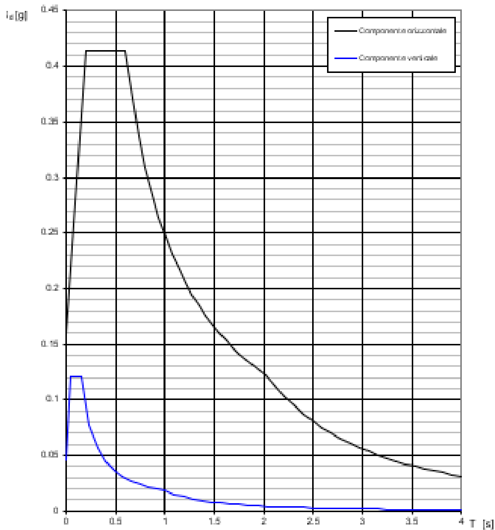
Figura 6-1 - Spettri di risposta di progetto sito specifici in componente verticale e orizzontale per lo SLV
