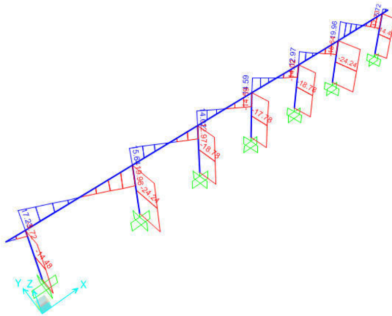
Figura 9-2 –Sforzo di Taglio [KN]
