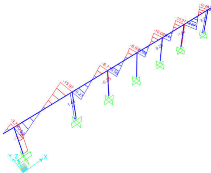
Figura 9-3 –Sforzo di Taglio [KN]
