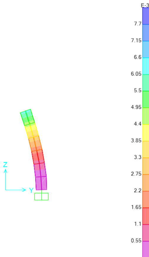
Figura 9-6 – Configurazione deformata
