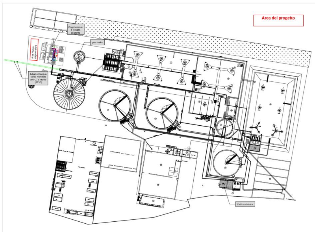
Figura 6.3 – Schema dell'impianto Trattamento Acque in rosso l'area dove sarà ubicato il container
