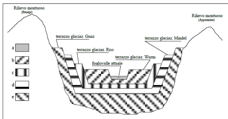
Figura 7.24 – Schema semplificato della struttura geologica di una valle di tipo Padano
