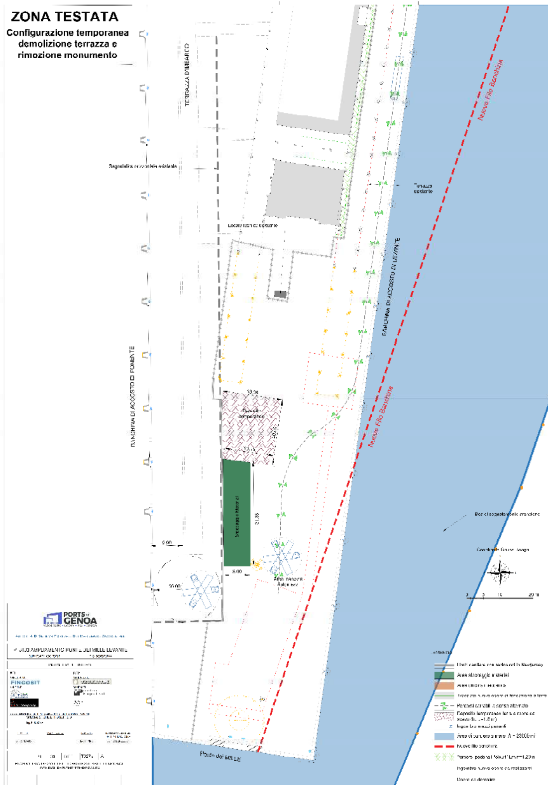
Figura 2 Planimetria di cantiere – logistica e aree funzionali configurazione temporanea
