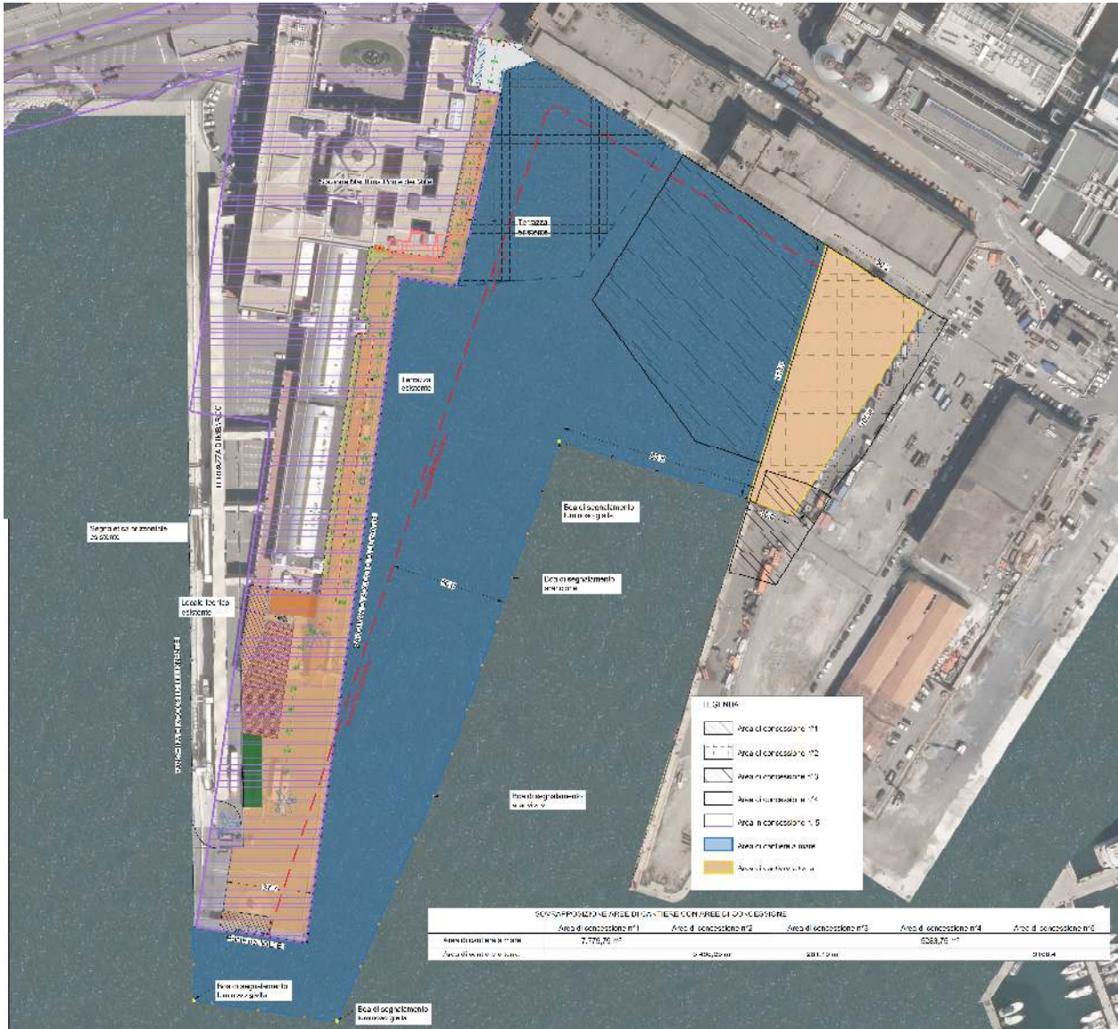
Figura 1 Planimetria di cantiere - Viabilità
