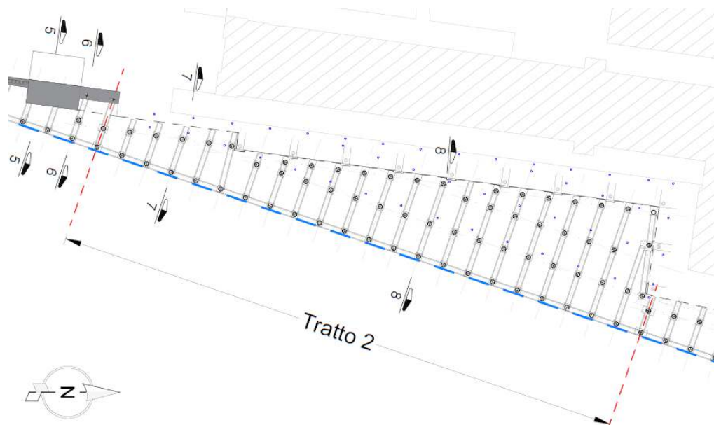
Figura 13 - Planimetria di intervento – Tratto 2
