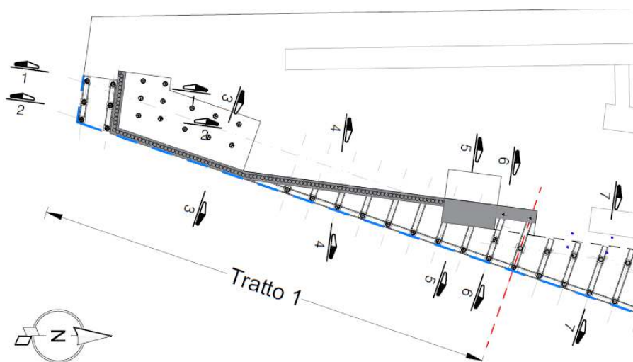
Figura 11 - Planimetria di intervento – Tratto 1
