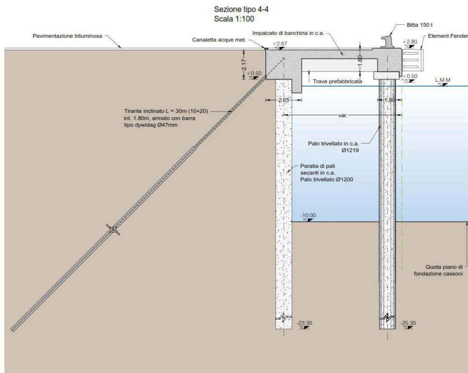
Figura 12 – sezione tipo d'intervento
