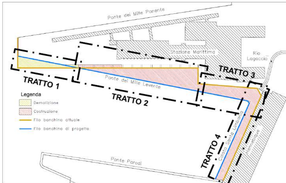
Figura 10 - Sovrapposizione stato attuale/progetto
