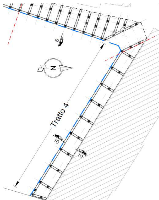
Fig. 16 - Planimetria di intervento – Tratto 4
