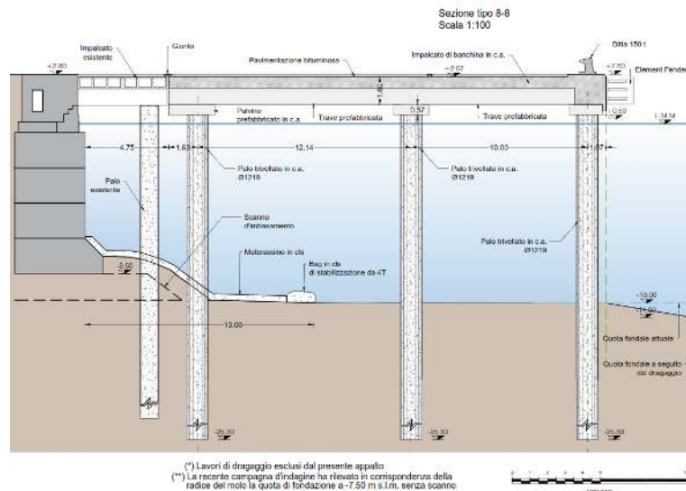
Figura 14 – sezione tipo d'intervento
