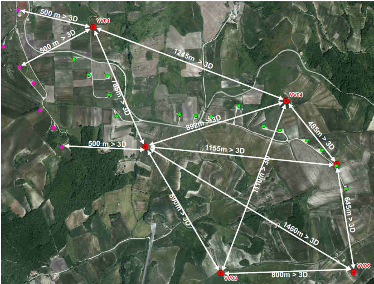
Figura 11: Schema layout con indicazione delle interdistanze tra le tribune di progetto
