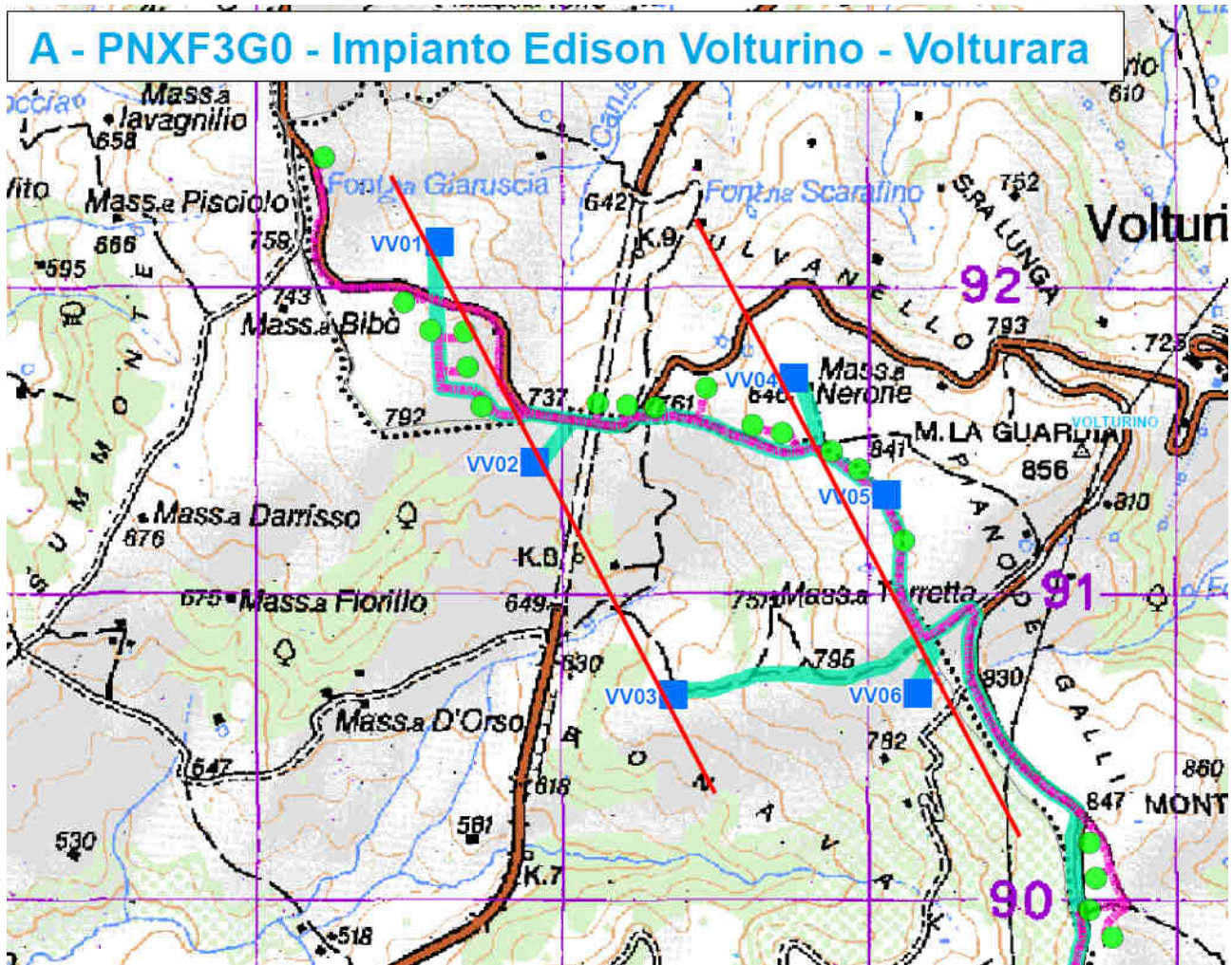
Figura 24: Schema impianto lineare (quadrati blu: nuovo impianto; cerchi verdi: wtg da smantellare)
