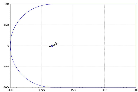
Figura 5.1 - Dominio di calcolo
