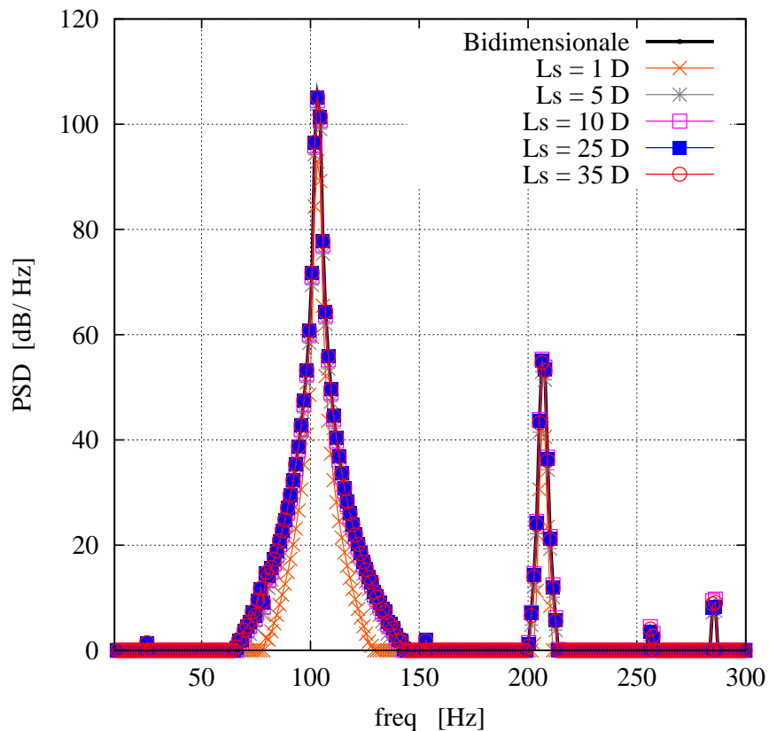
Figura 5.3 Sensibilità dello spettro al crescere della lunghezza spanwise simulata
