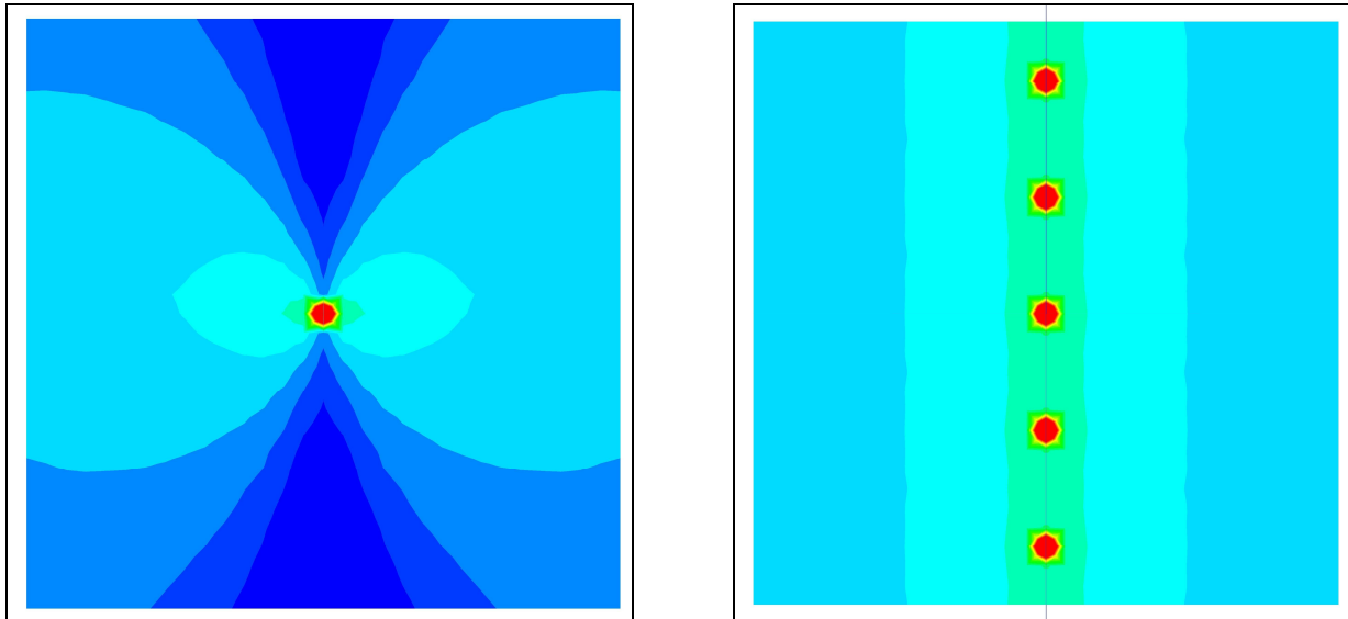
Figura 5.10 Effetto dell'introduzione di valori di direttività per una sorgente lineare, Piano XY – Piano XZ
