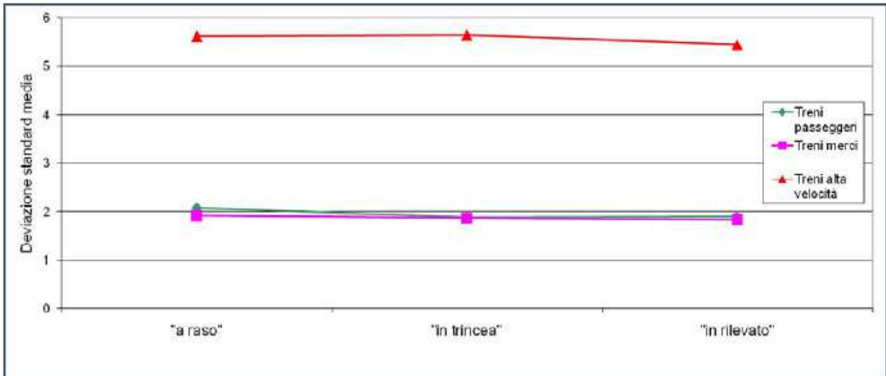
Figura 3.27 Deviazione standard media per categoria di treno nelle configurazioni del tracciato "a raso", "in trincea" e "in rilevato"
