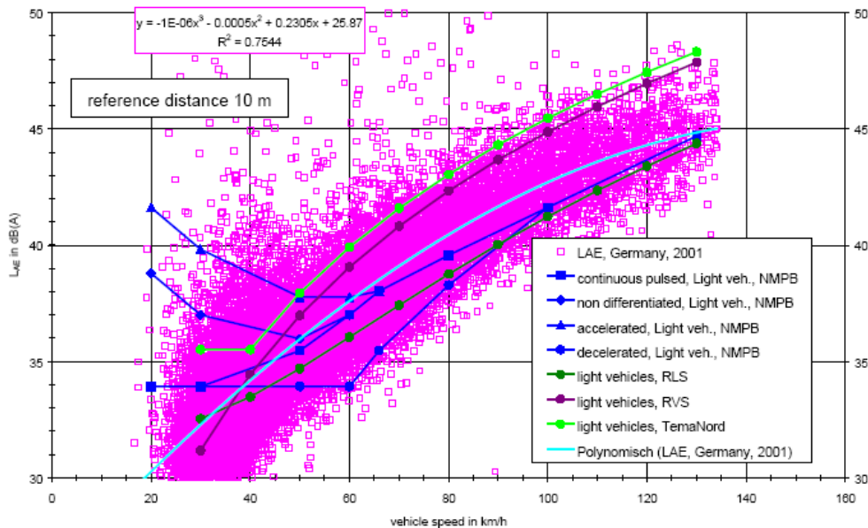
Figura 3.2 Valori di emissione LAE in funzione della velocità per veicoli leggeri
