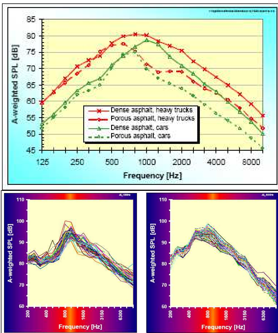
Figura 3.17 Spettri di rumore per veicoli leggeri e pesanti su pavimentazioni in asfalto tradizionale (sx) e drenante (dx)
