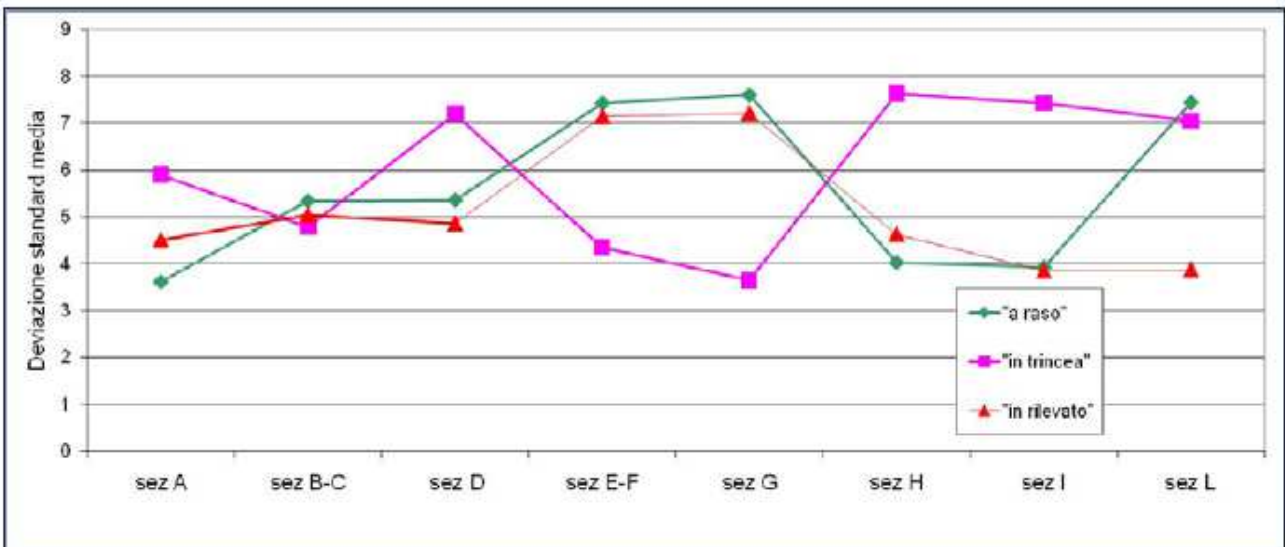
Figura 3.26 Deviazioni standard medie, calcolate per i treni ad alta velocità, lungo le sezioni del tracciato nei casi di linea "a raso", "in trincea" e "in rilevato"
