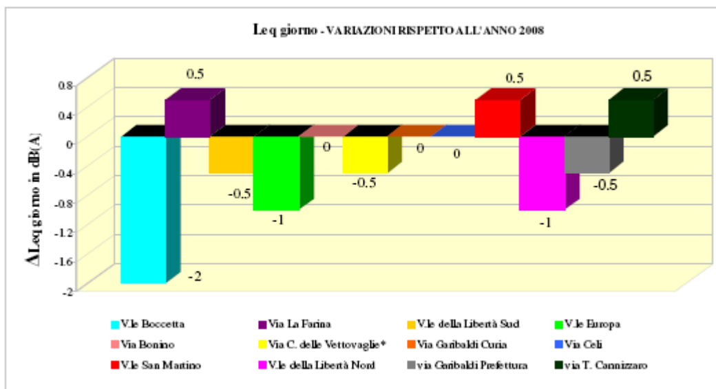
Figura 2.32 Sintesi Livelli diurni nei viali cittadini
