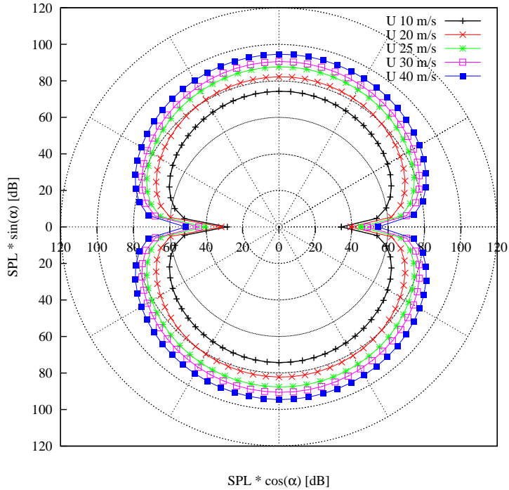
Figura 5.5 Direttività dell'emissione acustica
