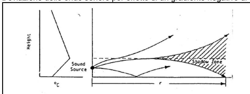
Deviazione delle onde sonore in presenza di un'inversione del gradiente di T
