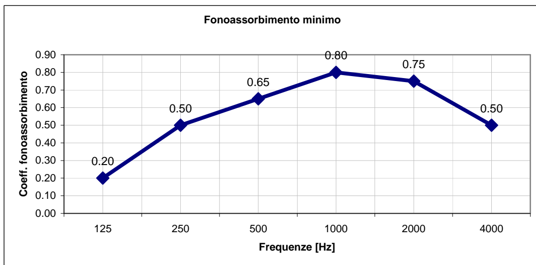
Figura 3.18 Coefficienti di fonoassorbimento minimi barriere antirumore (DMA 29.11.2000)
