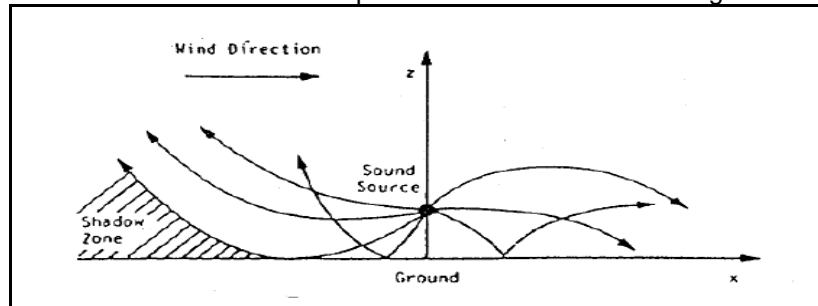
Effetto congiunto vento e gradiente di temperatura sulla deviazione delle onde sonore
