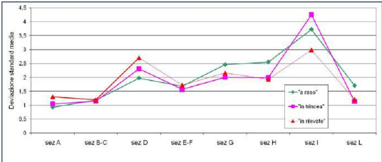
Figura 3.25 Deviazioni standard medie, calcolate per i treni passeggeri e merci, lungo le sezioni del tracciato nei casi di linea "a raso", "in trincea" e "in rilevato"
