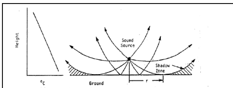
Deviazione delle onde sonore per effetto di un gradiente negativo di T
