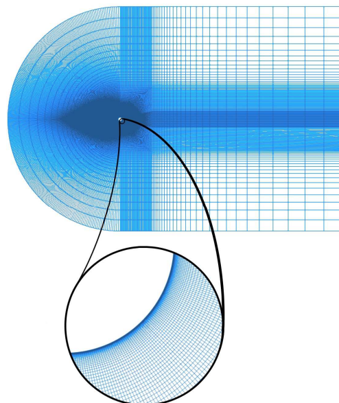
Figura 5.2 - Griglia di calcolo
