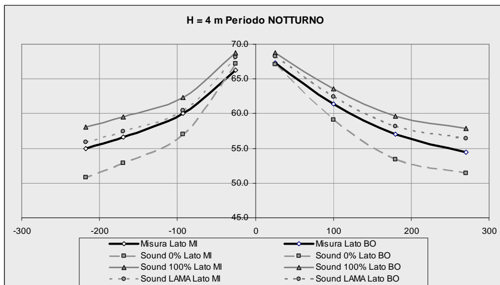
Figura 3.3 Confronto tra dati sperimentali e previsionali NMPB96 in periodo diurno e notturno per % di condizioni favorevoli 0-50-100 e locali (LAMA)
