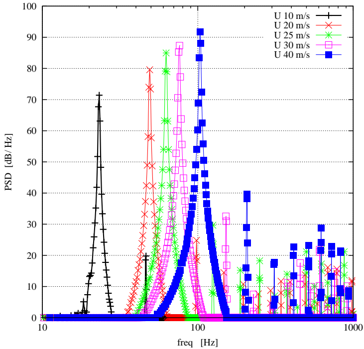
Figura 5.6 Spettri acustici valutati a 90°
