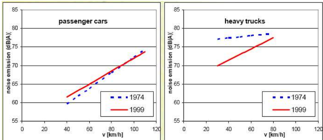
Figura 3.7 Emissioni di rumore in funzione della velocità, veicoli leggeri e pesanti
