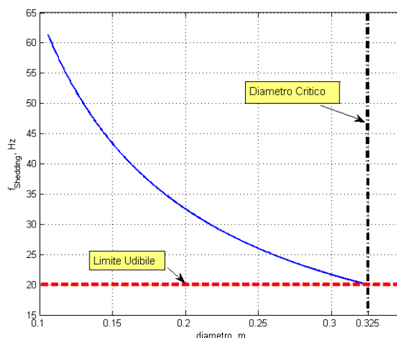
Figura 5.9 Frequenza shedding stimata per U=25\text{m/s} e St=0.26
