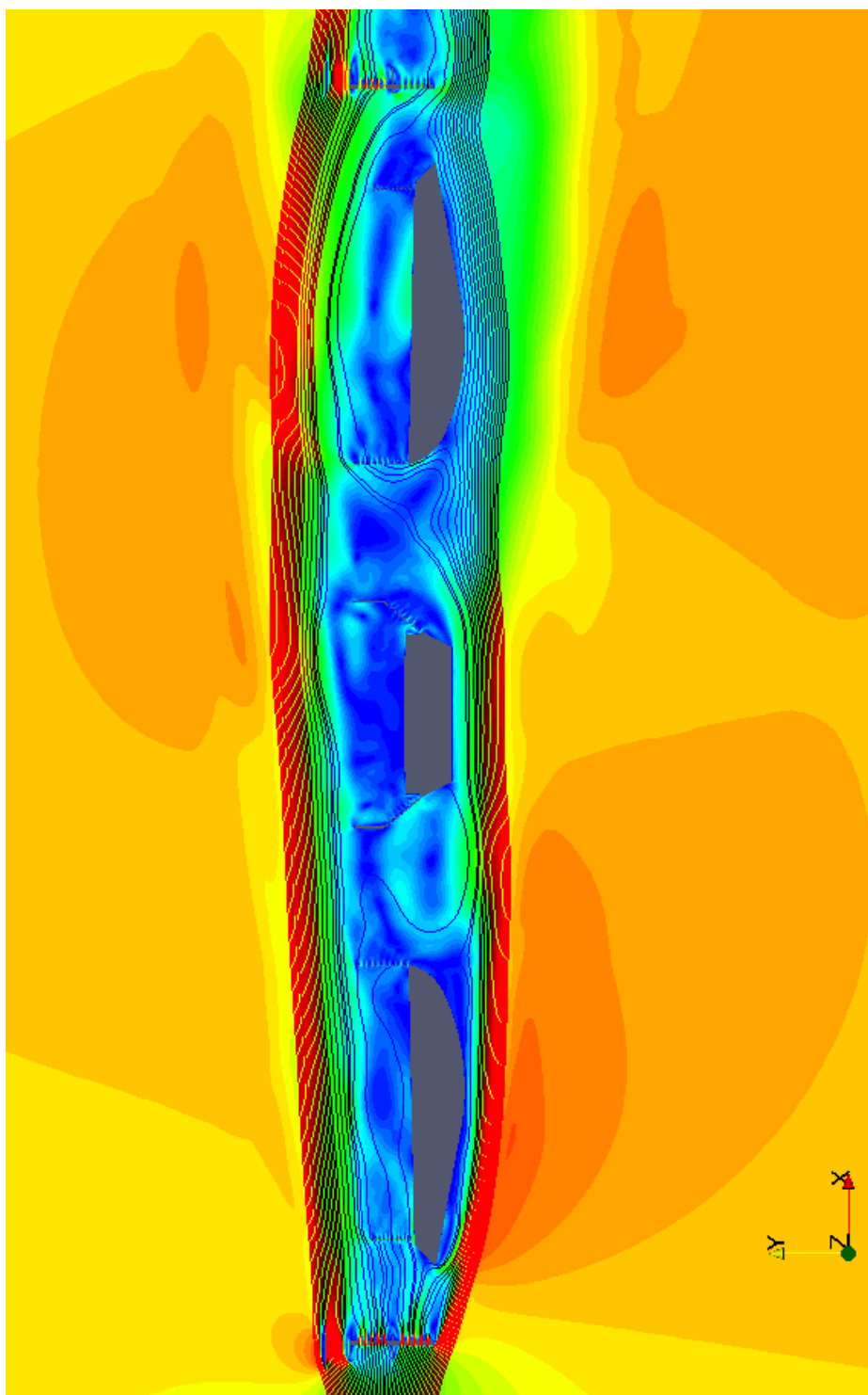
Figura 5.8 Linee di corrente del campo medio in prossimità dell'impalcato
