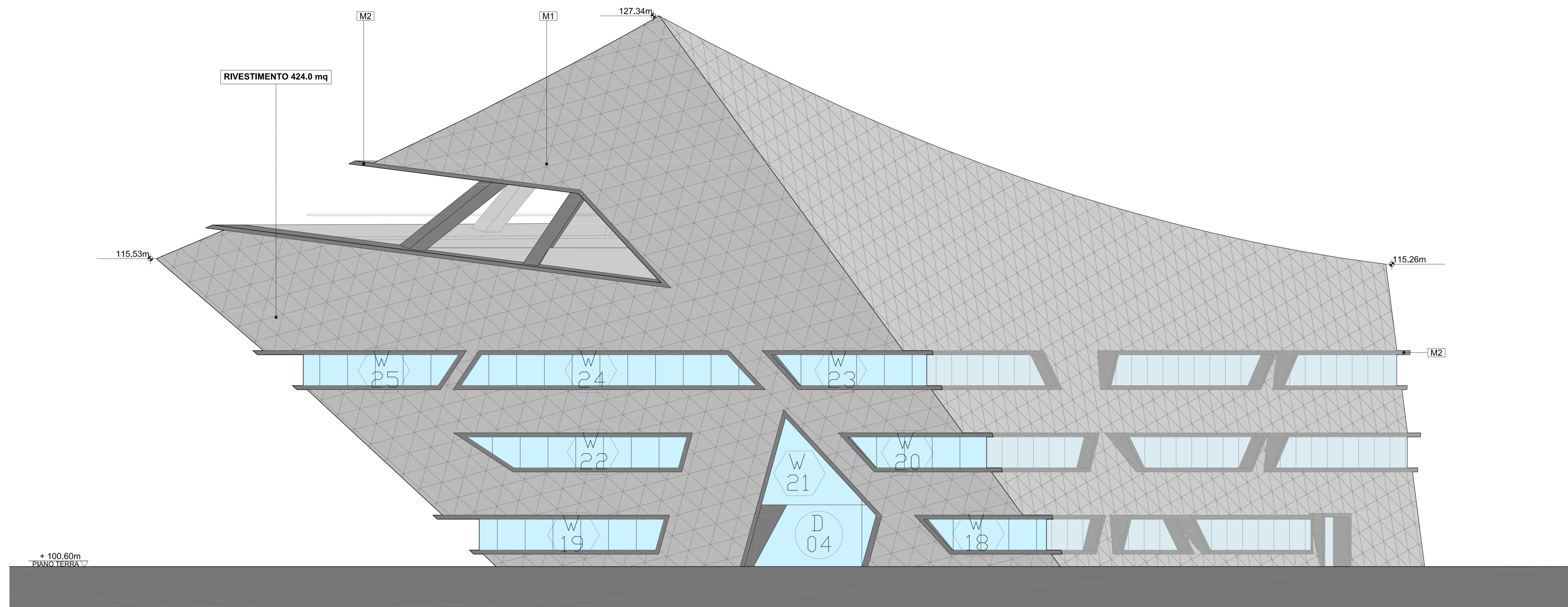
01 PROSPETTO OVEST SCALA 1:100
