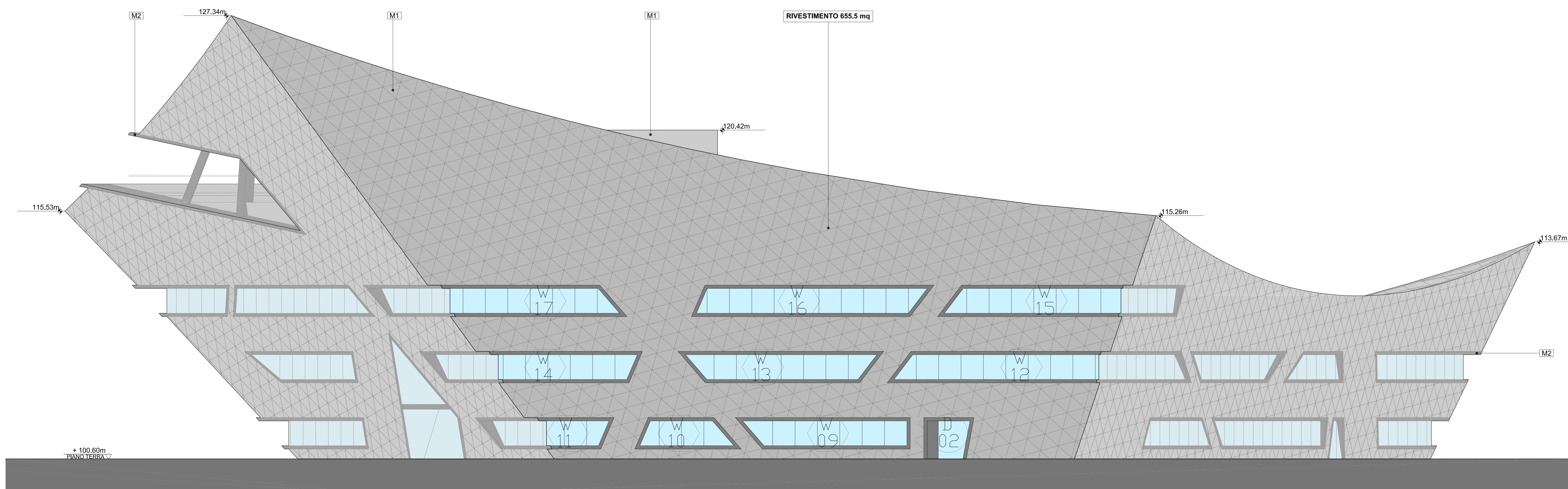
02 PROSPETTO SUD-OVEST SCALA 1:100
