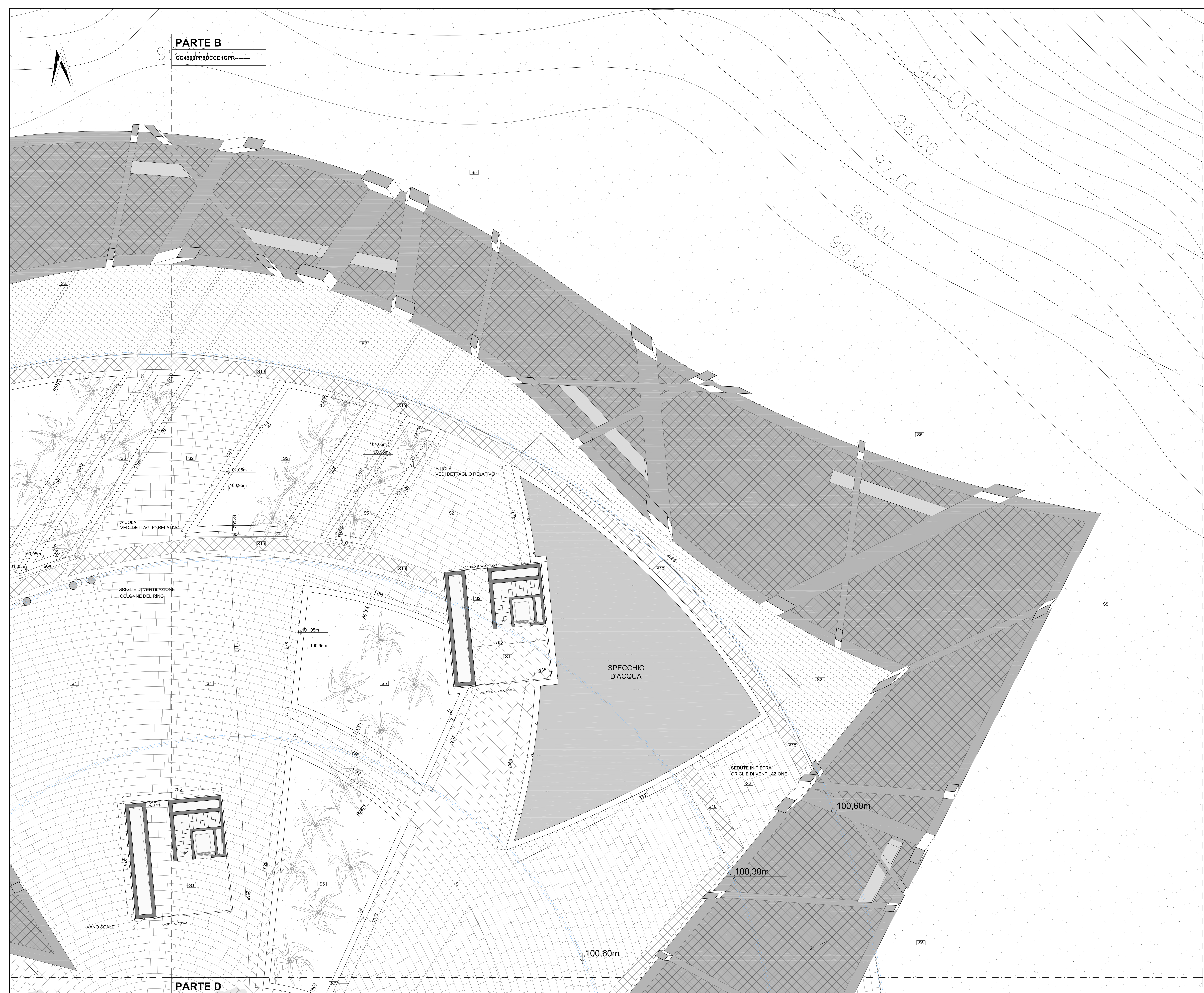
01 ARCADE : PIANTE A LIVELLO (quota 100.60) - Tavola 2/4 1:100
