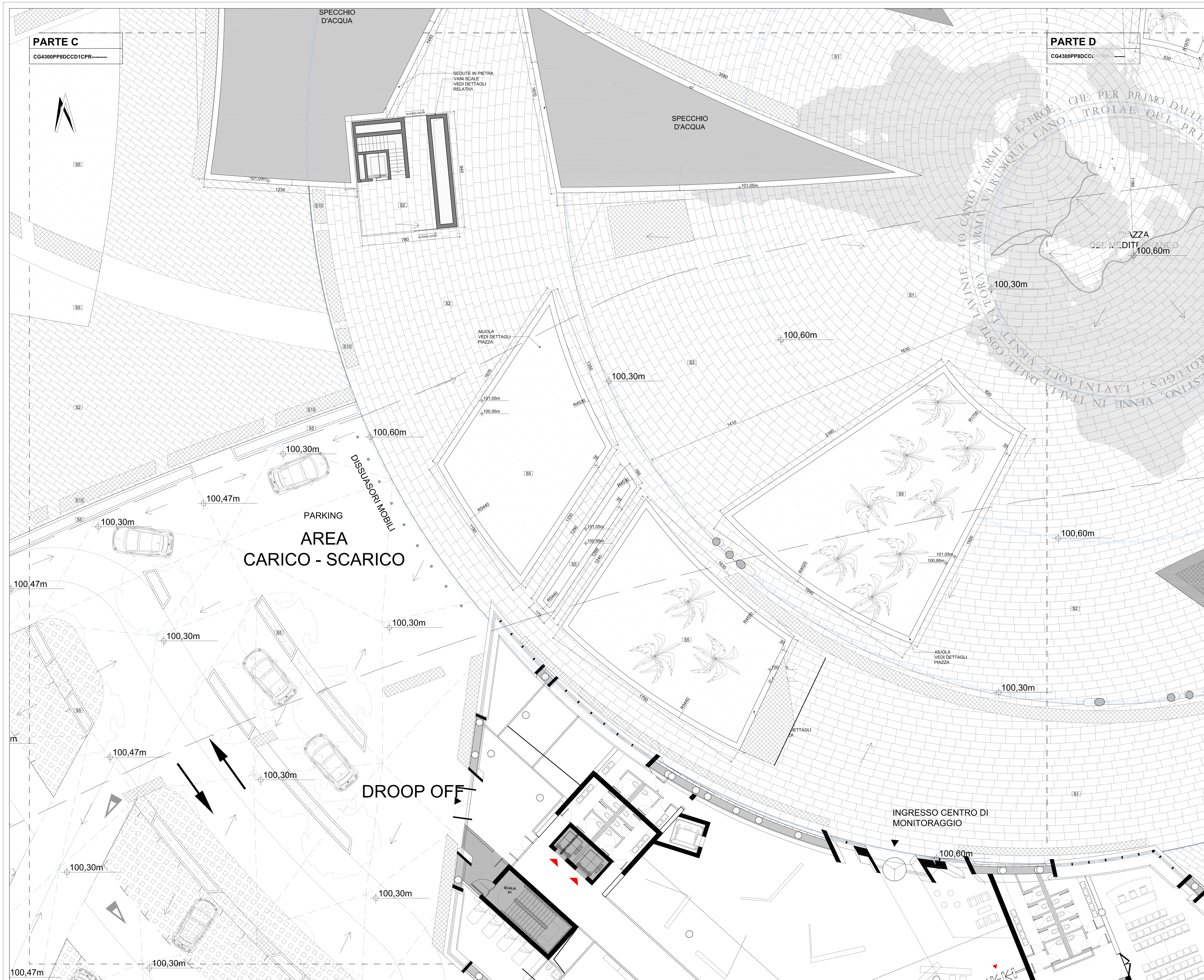
01 ARCADE : PIANTA A LIVELLO (quota 100.60) - Tavola 3/4 1:100
