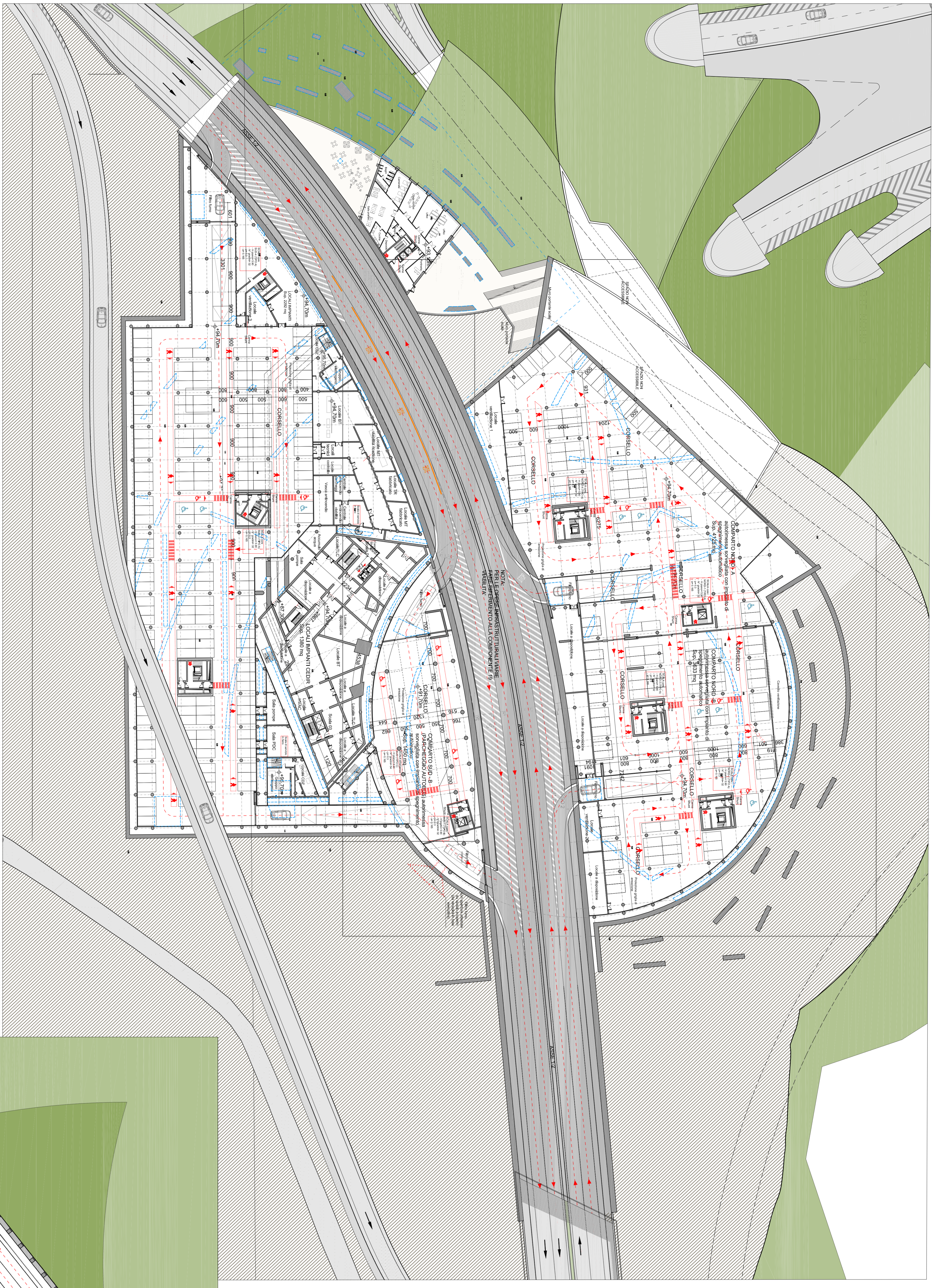
01 PLANIMETRIA GENERALE PARCHEGGIO INTERRATI (quota 94.70) 1:500
