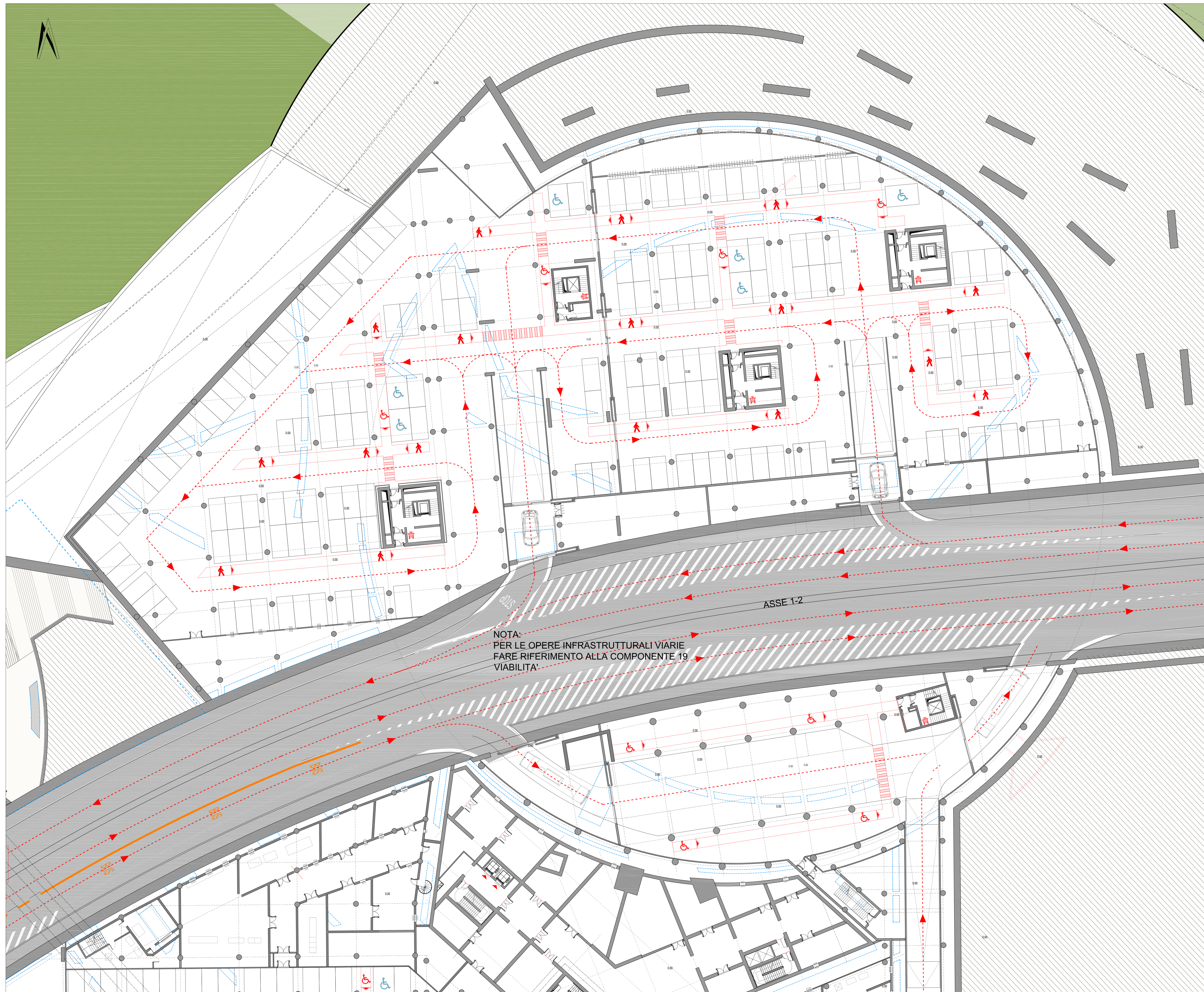
01 PIANTA PARCHEGGIO INTERRATO L-1 COMPARTO NORD (quota 94.70 m)
