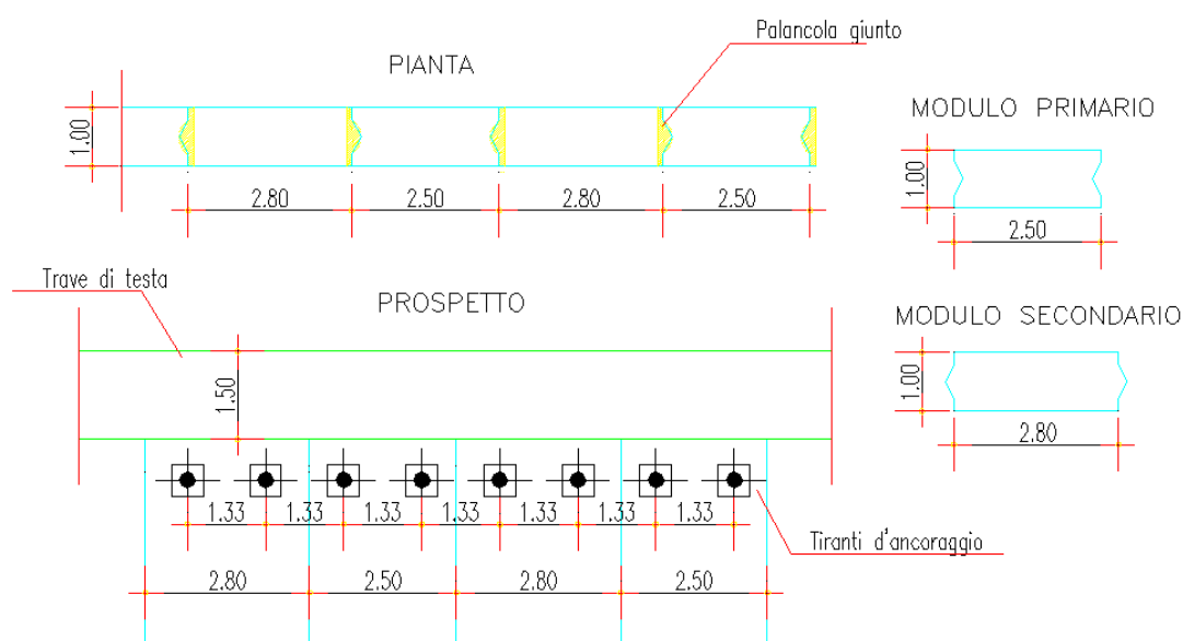
Figura 1.1: Dettaglio pannelli
