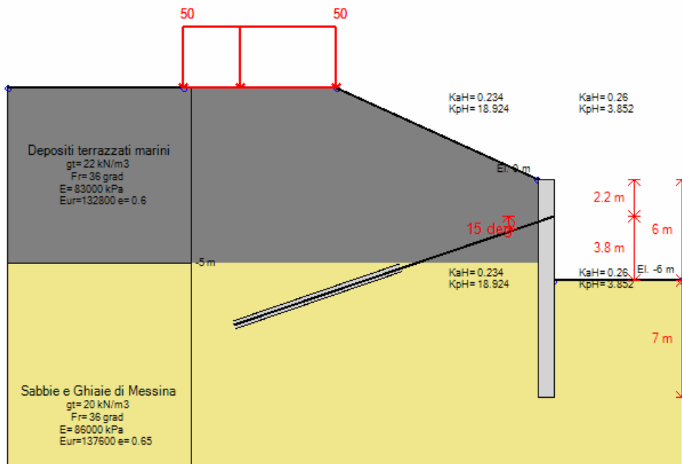
Stage 3 – Scavo a quota -6.00 m
