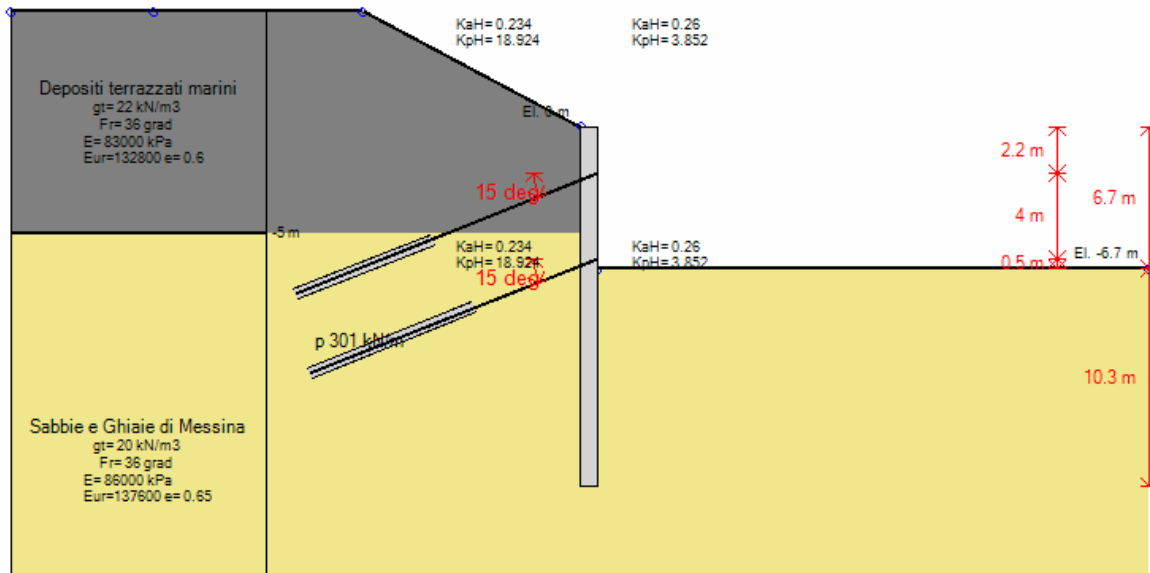
Stage 4 –Inserimento tirante a quota -6.20 m
