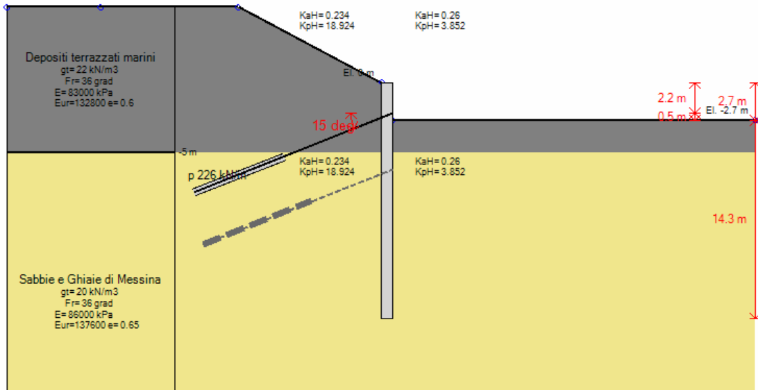
Stage 2 – Inserimento tirante a quota -2.20 m
