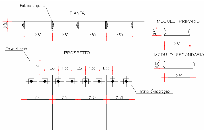
Fig. 4.1 – Dettaglio dei diaframmi
