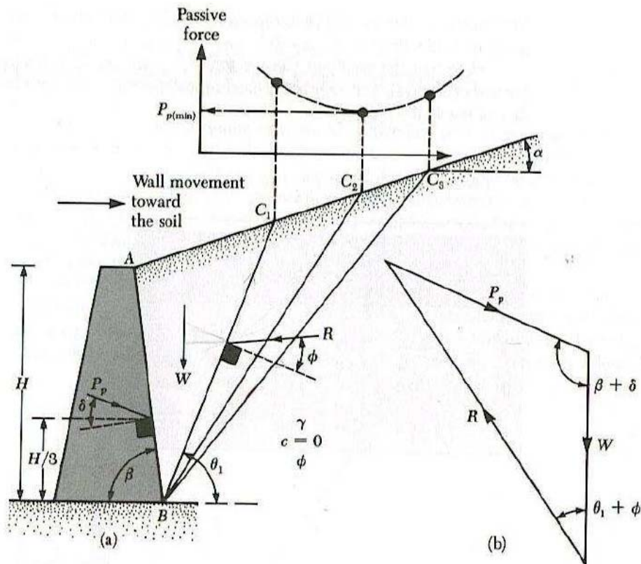
Figura 10.2: Ricerca del cuneo di spinta passiva col metodo dei cunei
