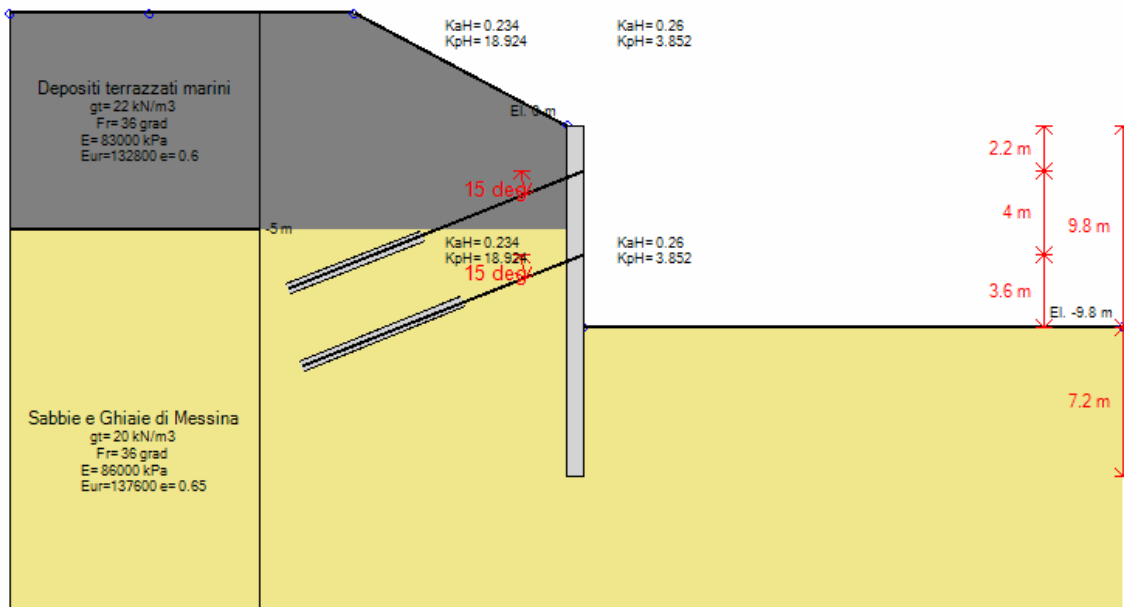
Stage 5 –Scavo a quota -9.80 m
