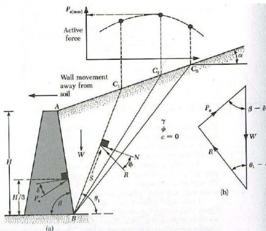
Figura 10.1: Ricerca del cuneo di spinta attiva col metodo dei cunei
