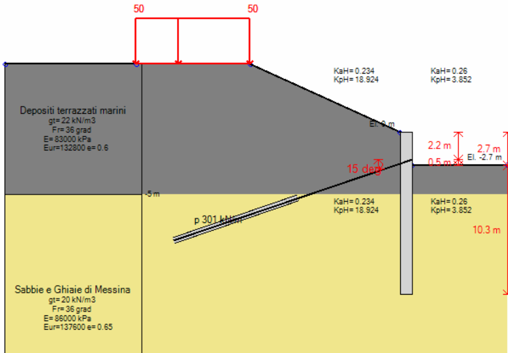
Stage 2 – Inserimento tirante a quota -2.20 m
