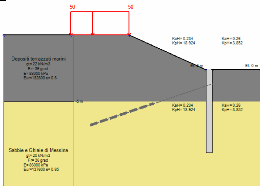
Stage 0 – Infissione
