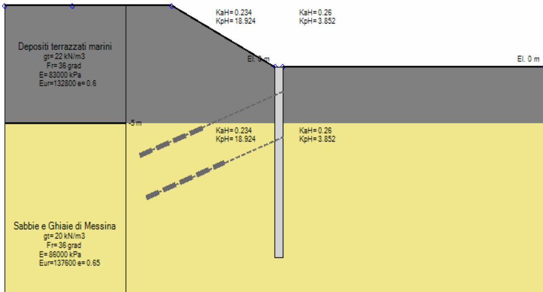
Stage 0 – Infissione
