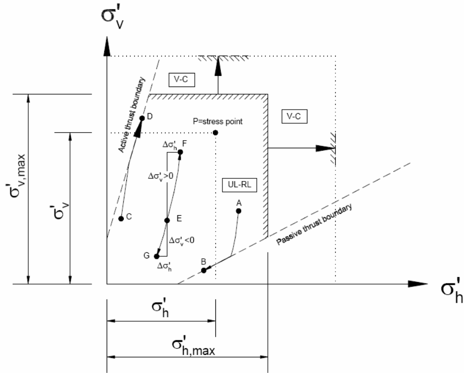
Figura 10.3: Modello per terreni granulari
