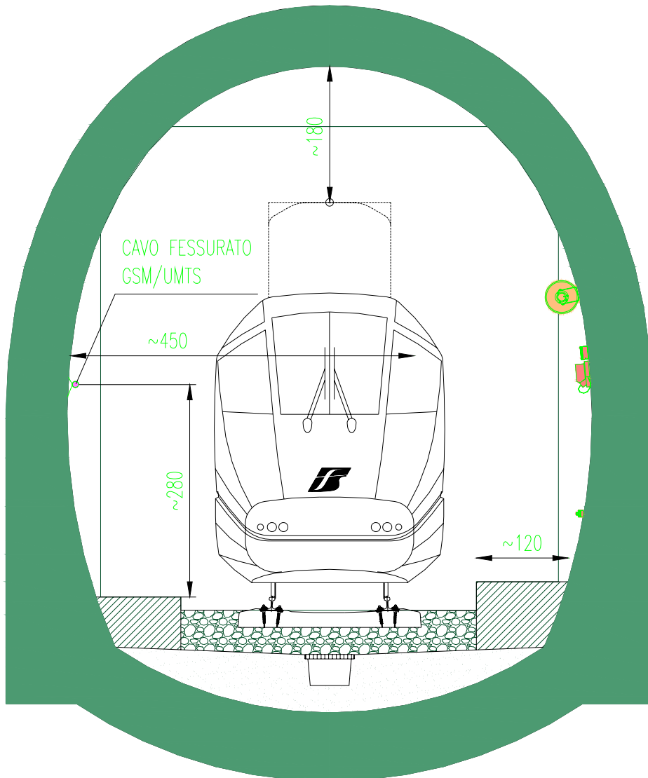
Sezione trasversale tipica della galleria ferroviaria Bolano
