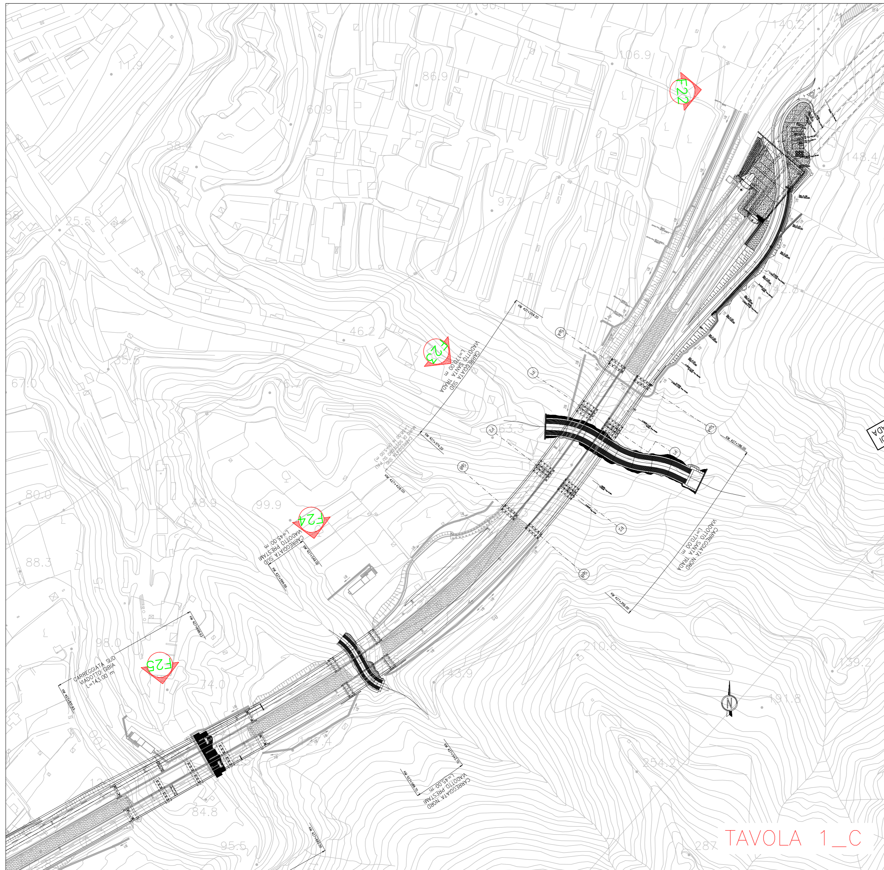
F25 - VIADOTTO GIBIA
