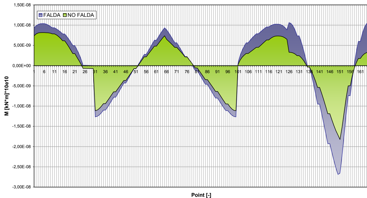
CONFRONTO MOMENTI RIVESTIMENTO DEFINITIVO - FASE DI CALCOLO 7
