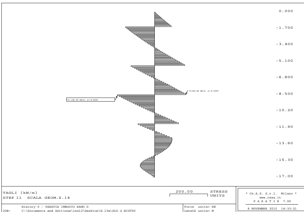
Figura 32 - Combinazione A2+M2 (SLV): Sollecitazioni di taglio agenti sul palo
