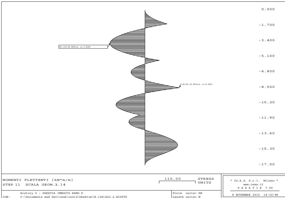
Figura 31 - Combinazione A2+M2 (SLV): Momento flettente agente sul palo
