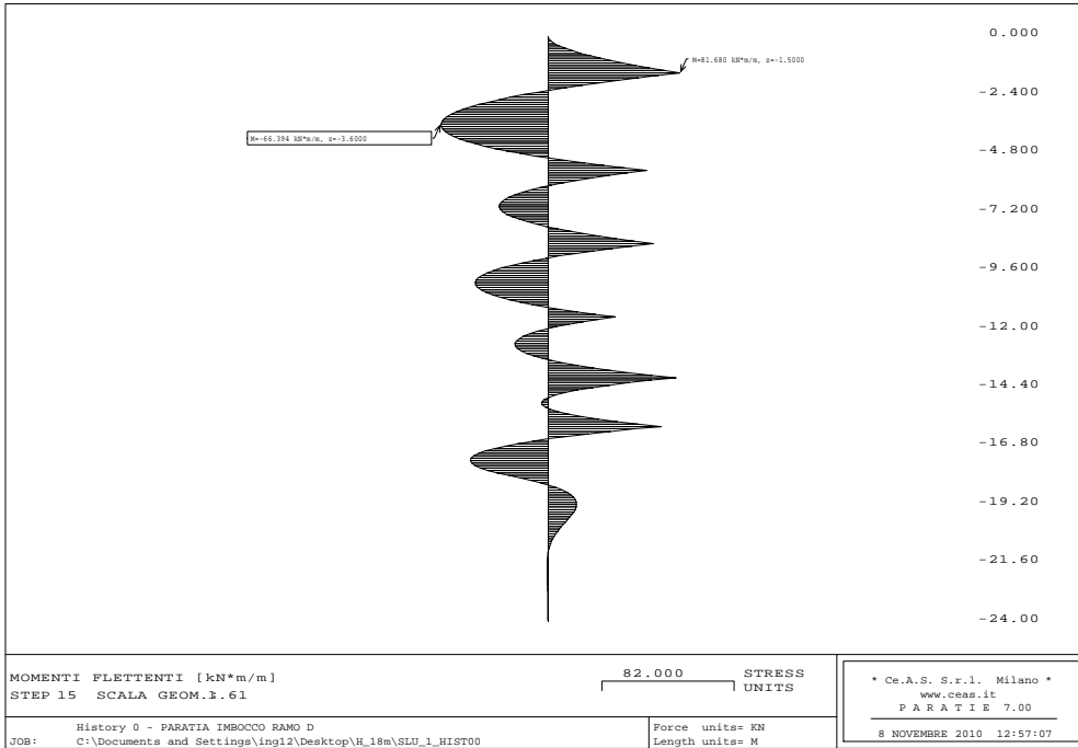
Figura 27 - Combinazione A1+M1 (SLV): Momento flettente agente sul palo
