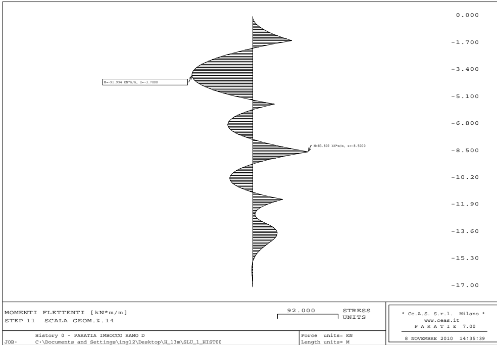
Figura 35 - Combinazione A1+M1 (SLV): Momento flettente agente sul palo
