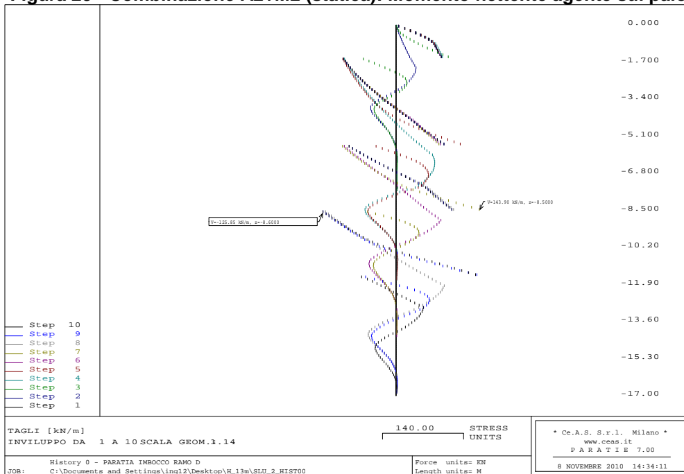
Figura 30 - Combinazione A2+M2 (statica): Sollecitazioni di taglio agenti sul palo
