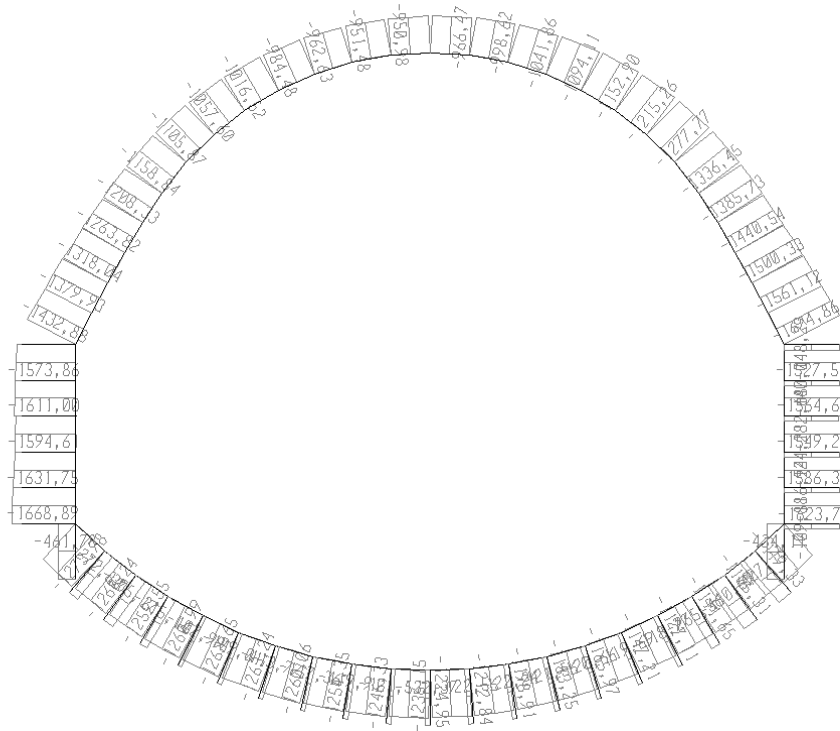
Figura 57 - COMBINAZIONE SLU (statica) Sforzo Assiale
