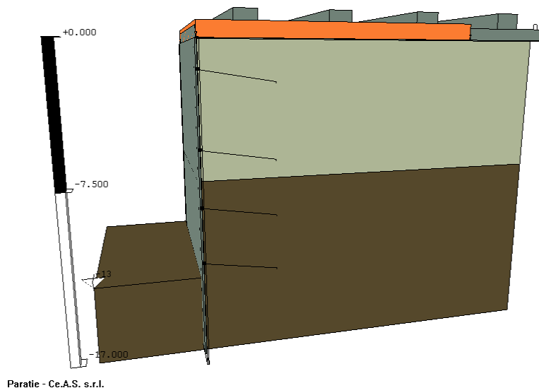
Figura 10 - Modello di calcolo per altezza fuori terra 13.0 m (sezione 2)
