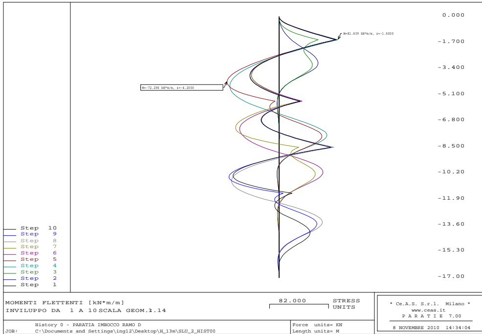
Figura 29 - Combinazione A2+M2 (statica): Momento flettente agente sul palo
