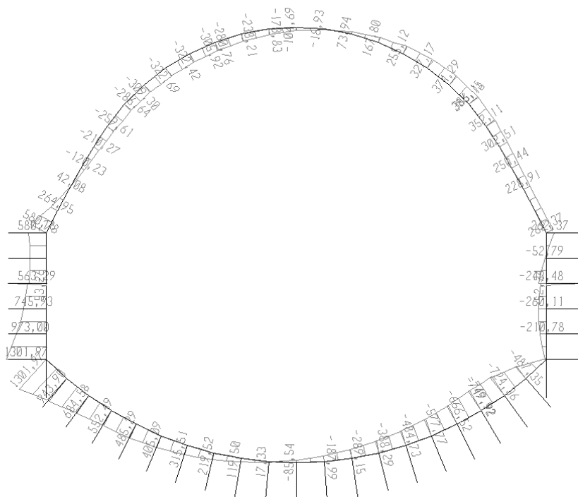
Figura 56 - COMBINAZIONE SLU (statica) Momento flettente
