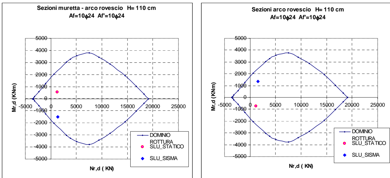
Figura 62 - Combinazione SLU statico e SLV : domini di resistenza delle sezioni oggetto di verifica
