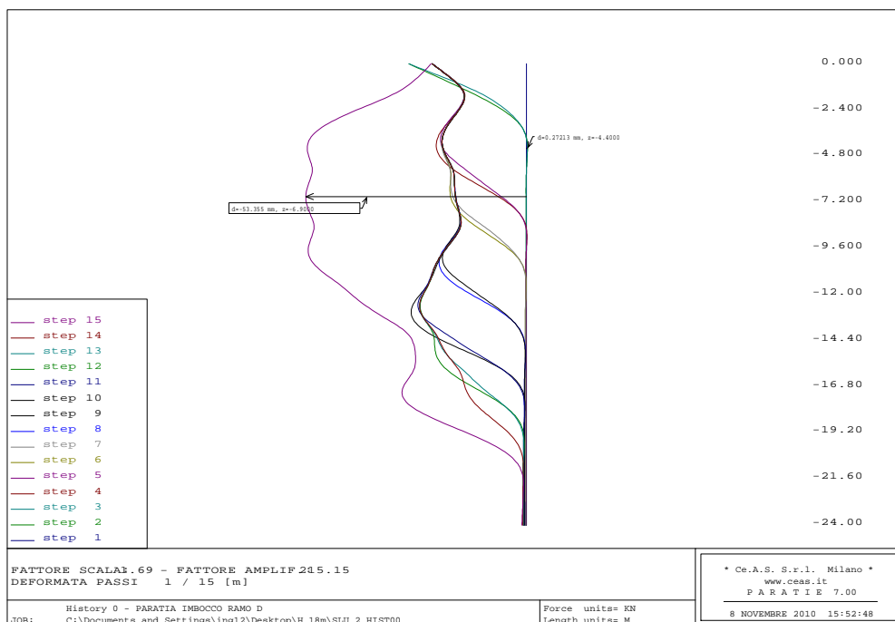
Figura 38 - Sezione di calcolo 1: deformata paratia - combinazione A2+M2
