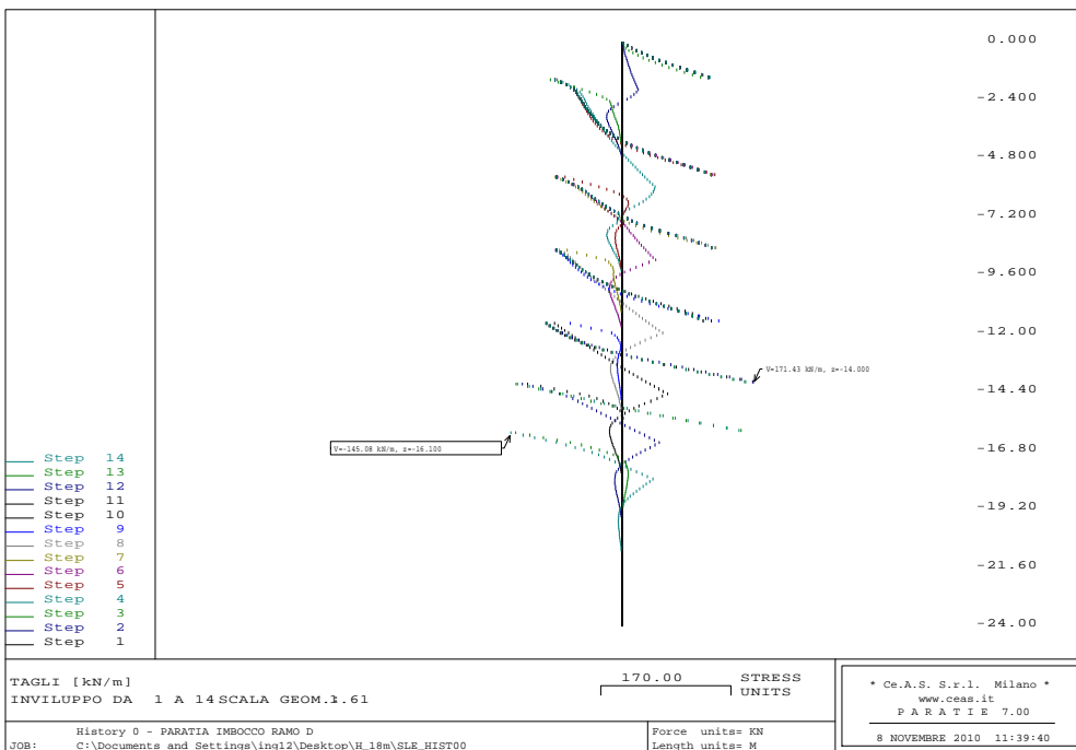
Figura 12 - Combinazione E1+E2 ( SLE) Sollecitazioni di taglio agenti sul palo
