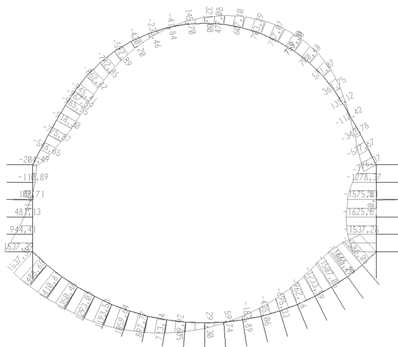
Figura 59 - COMBINAZIONE SLU (SLV)- Momento flettente
