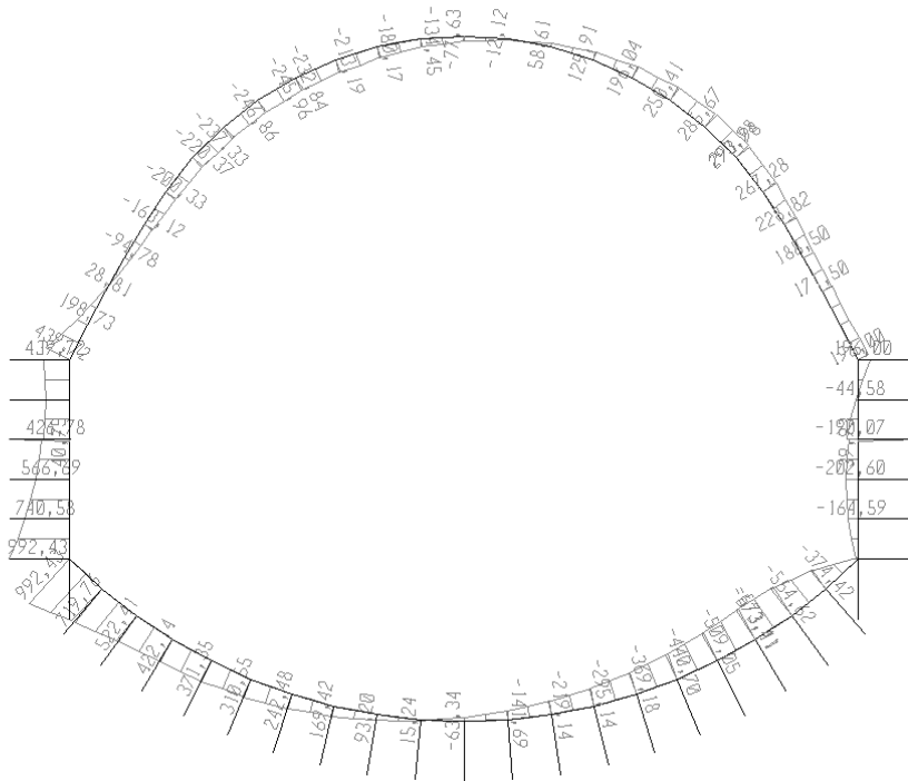
Figura 48 - COMBINAZIONE SLE- Momento flettente
