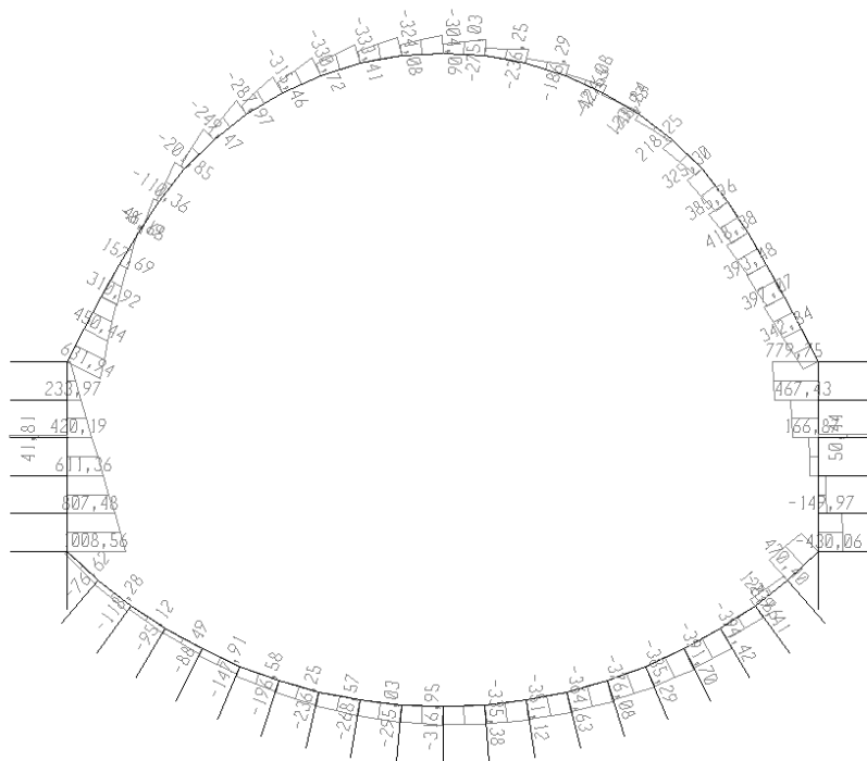
Figura 61 - COMBINAZIONE SLU (SLV) - Sforzo di Taglio
