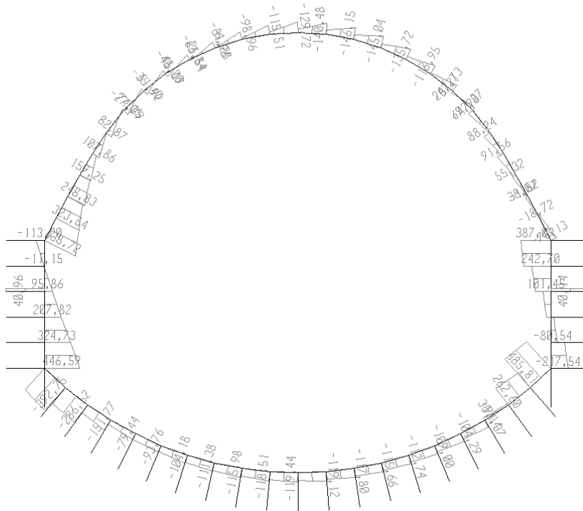
Figura 50 - COMBINAZIONE SLE- Sforzo di Taglio
