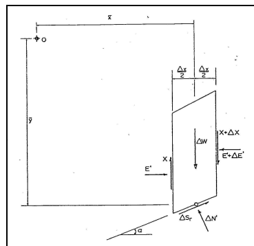
Figura 41 - Forze agenti sui conci
