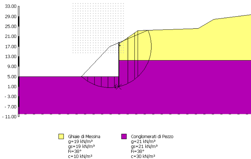
Figura 43 - Sezione calcolo 2– superfici di scorrimento critiche , valore minimo 1.35
