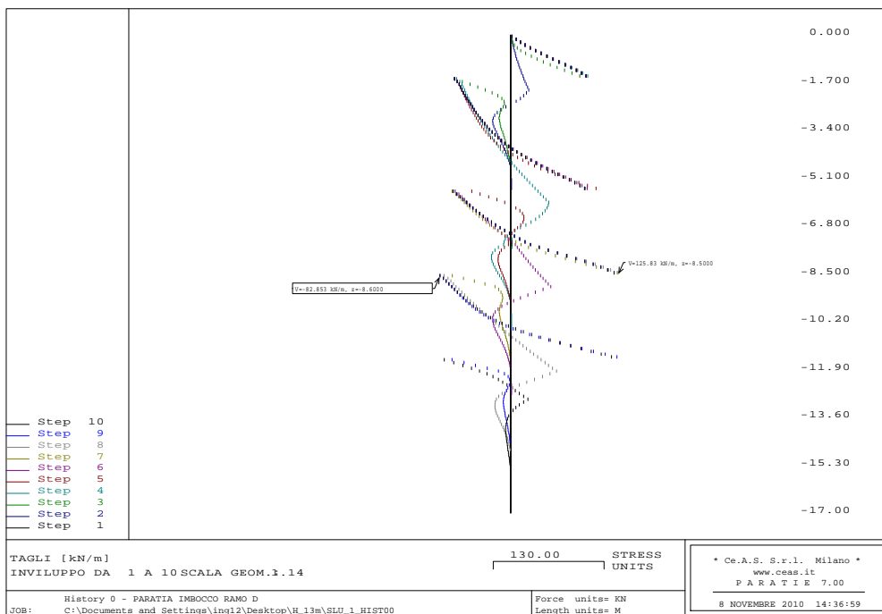
Figura 34 - Combinazione A1+M1 (statica): Sollecitazioni di taglio agenti sul palo
