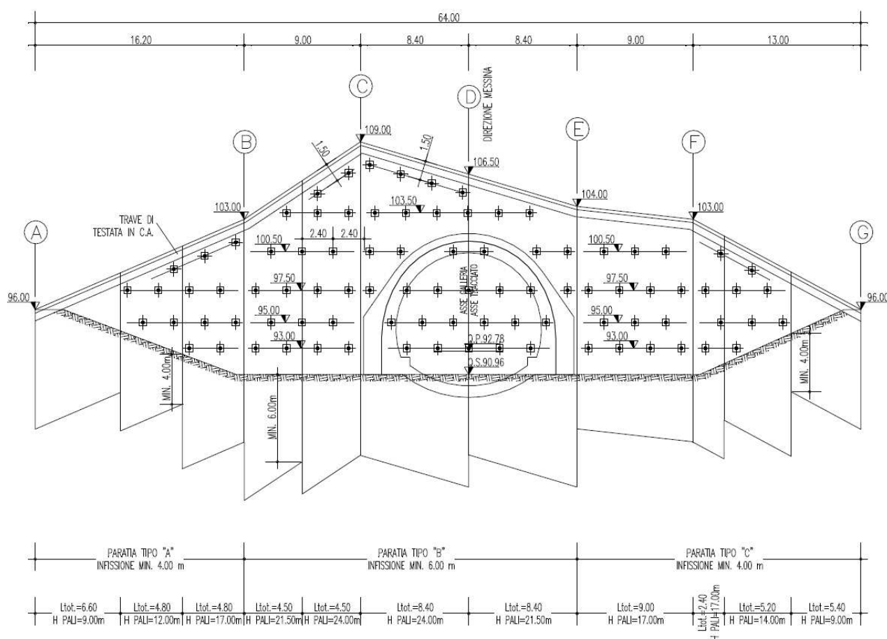
Figura 6 - Imbocco Balena Lato Messina Sviluppata Paratia
