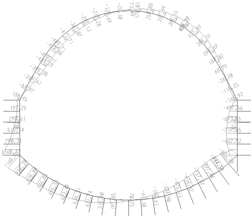
Figura 52 -COMBINAZIONE SLD- Momento flettente
