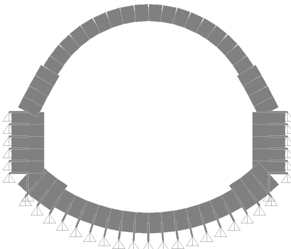
Figura 47 - Modellazione delle sezioni della galleria artificiale
