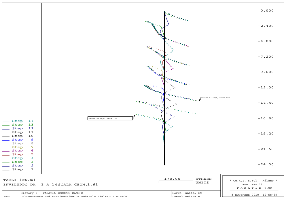
Figura 26 - Combinazione A1+M1 (Statica): Sollecitazioni di taglio agenti sul palo
