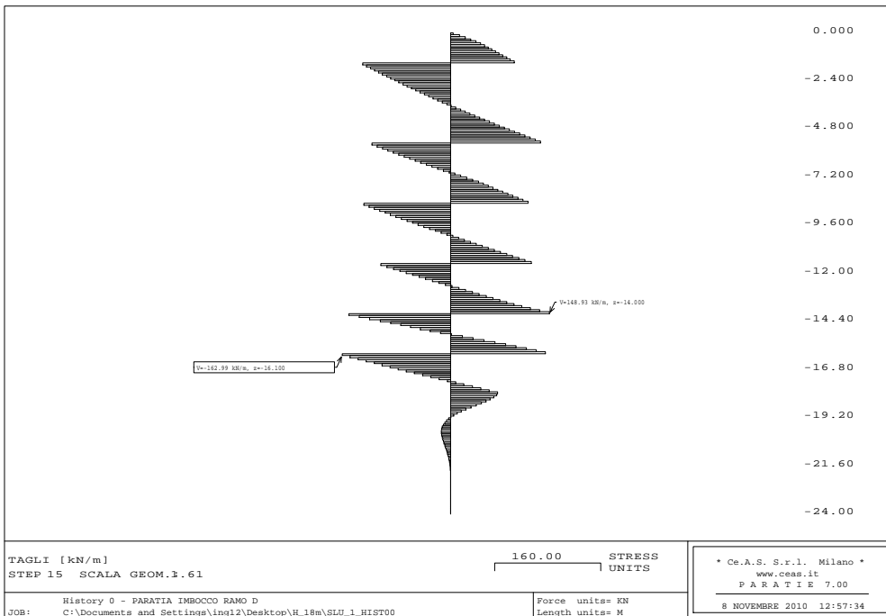
Figura 28 - Combinazione A2+M2 (SLV): Sollecitazioni di taglio agenti sul palo
