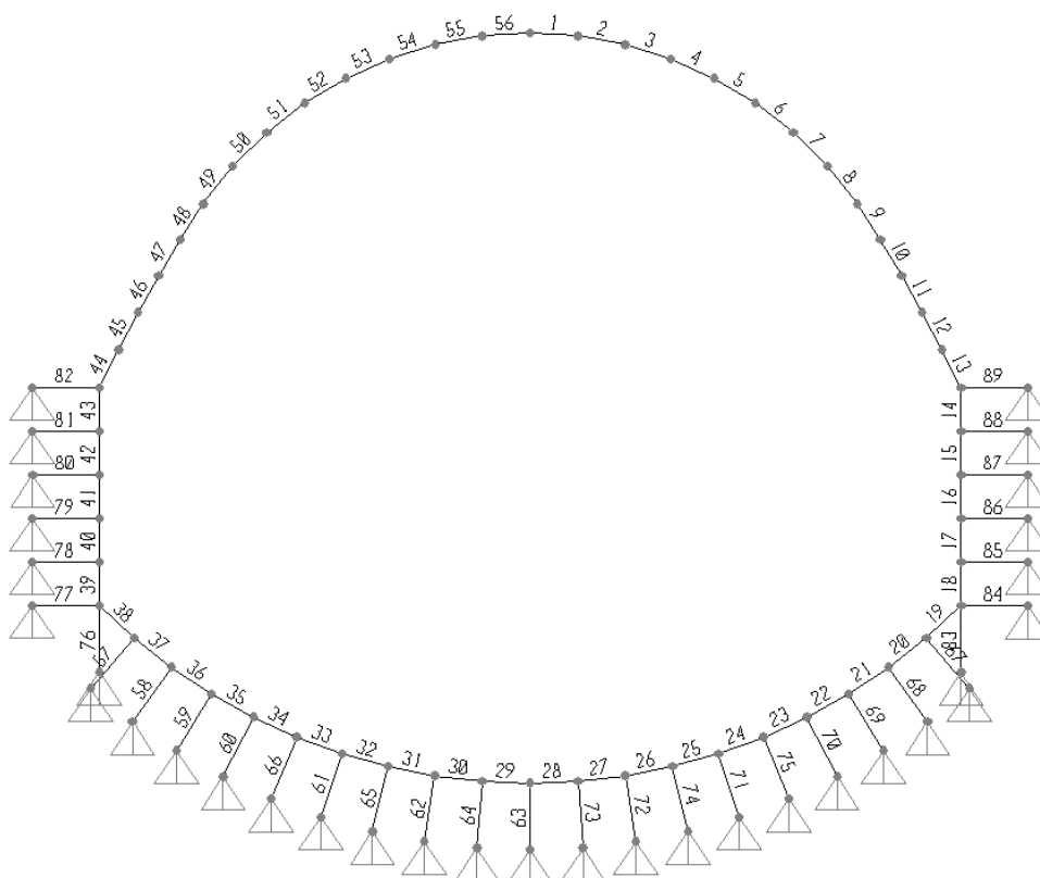
Figura 46 - Discretizzazione per elementi finiti tipo "Beam": numerazione elementi strutturali
