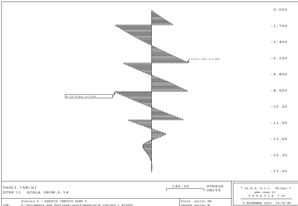
Figura 36 - Combinazione A1+M1 (SLV): Sollecitazioni di taglio agenti sul palo
