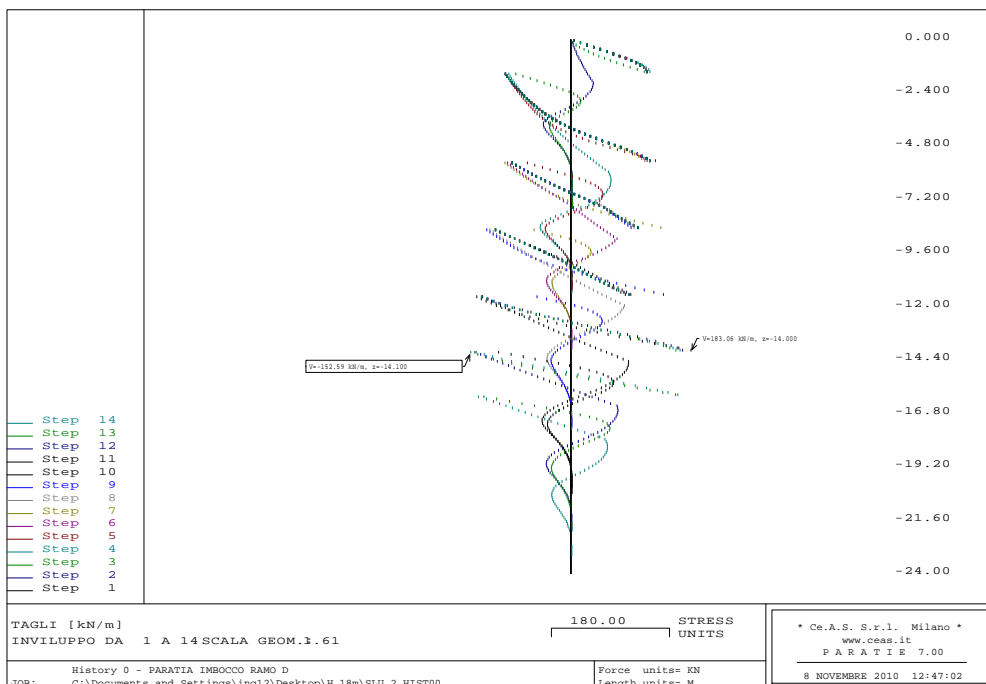
Figura 22 - Combinazione A2+M2 (Statica): Sollecitazioni di taglio agenti sul palo
