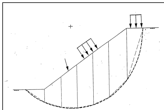
Figura 40 - Blocco di terreno instabile suddivisione in conci
