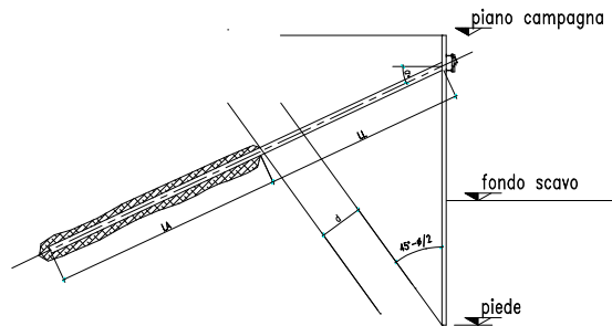
Figura 37 - Schema calcolo lunghezza libera del tirante
