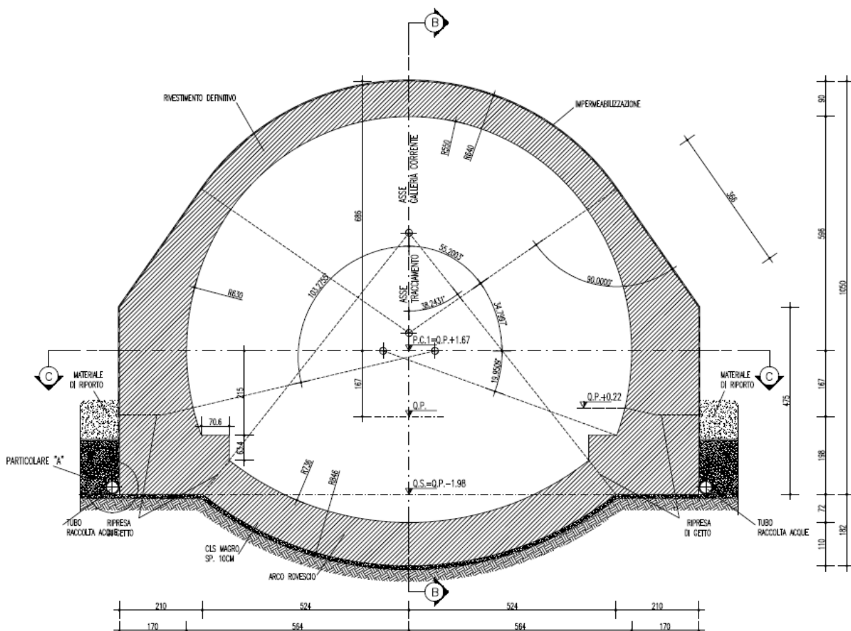
Figura 44 – Carpenteria tipologica galleria artificiale
