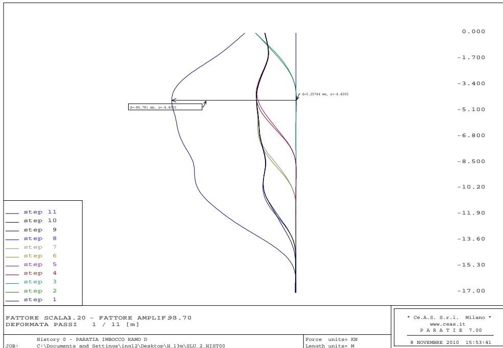
Figura 39 - Sezione di calcolo 2: deformata paratia - combinazione A2+M2
