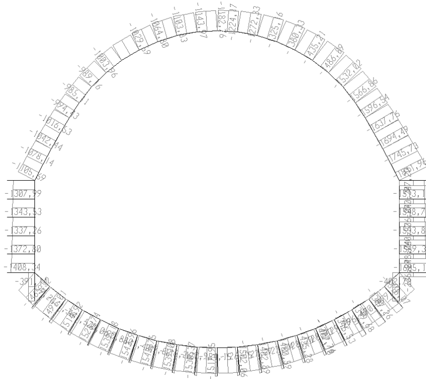
Figura 60 - COMBINAZIONE SLU (SLV) - Sforzo Normale
