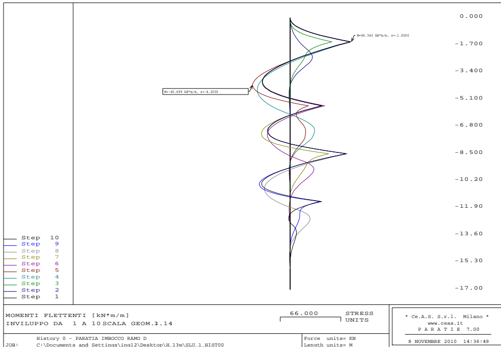
Figura 33 - Combinazione A1+M1 (statica): Momento flettente agente sul palo
