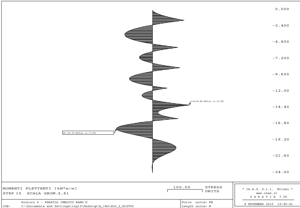
Figura 23 - Combinazione A2+M2 (SLV): Momento flettente agente sul palo
