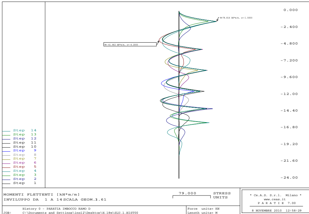
Figura 25 - Combinazione A1+M1 (Statica): Momento flettente agente sul palo
