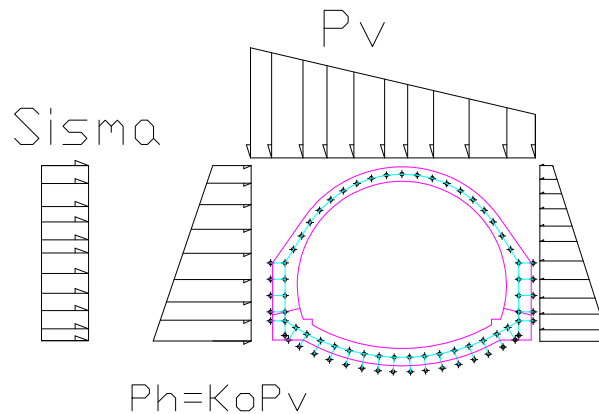
Figura 45 - Schema dei carichi applicati al modello numerico implementato
