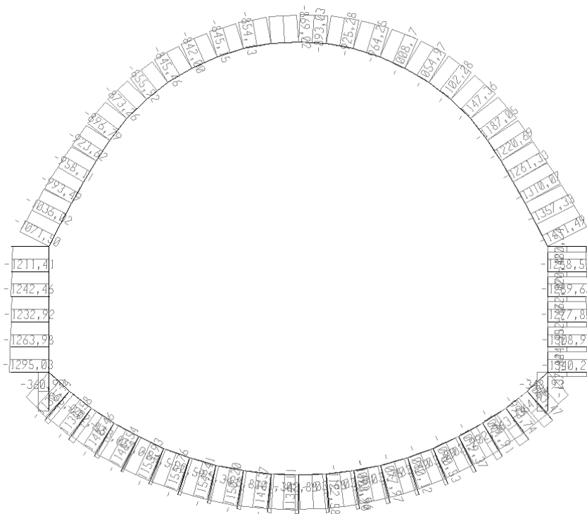
Figura 52 -COMBINAZIONE SLD- Momento flettente
