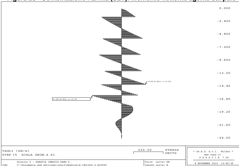
Figura 24 - Combinazione A2+M2 (SLV): Sollecitazioni di taglio agenti sul palo
