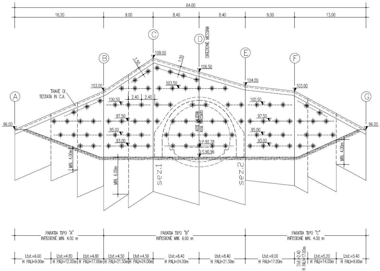
Figura 8 - Indicazione delle sezioni di calcolo
