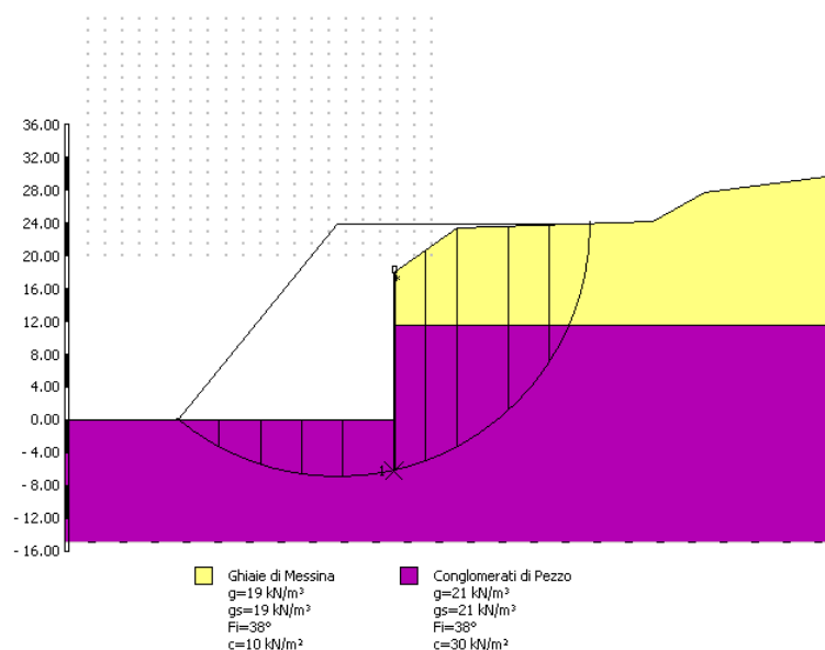
Figura 42 - Sezione di calcolo 1 – superfici di scorrimento critiche, valore minimo 1.45
