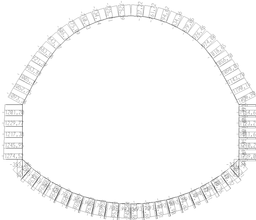
Figura 49 - COMBINAZIONE SLE- Sforzo Assiale
