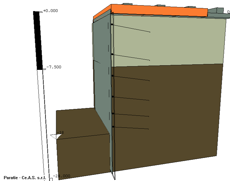
Figura 9 - Modello di calcolo per altezza fuori terra 18.0 m (sezione 1)
