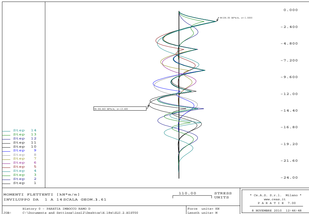
Figura 21 - Combinazione A2+M2 (Statica): Momento flettente agente sul palo
