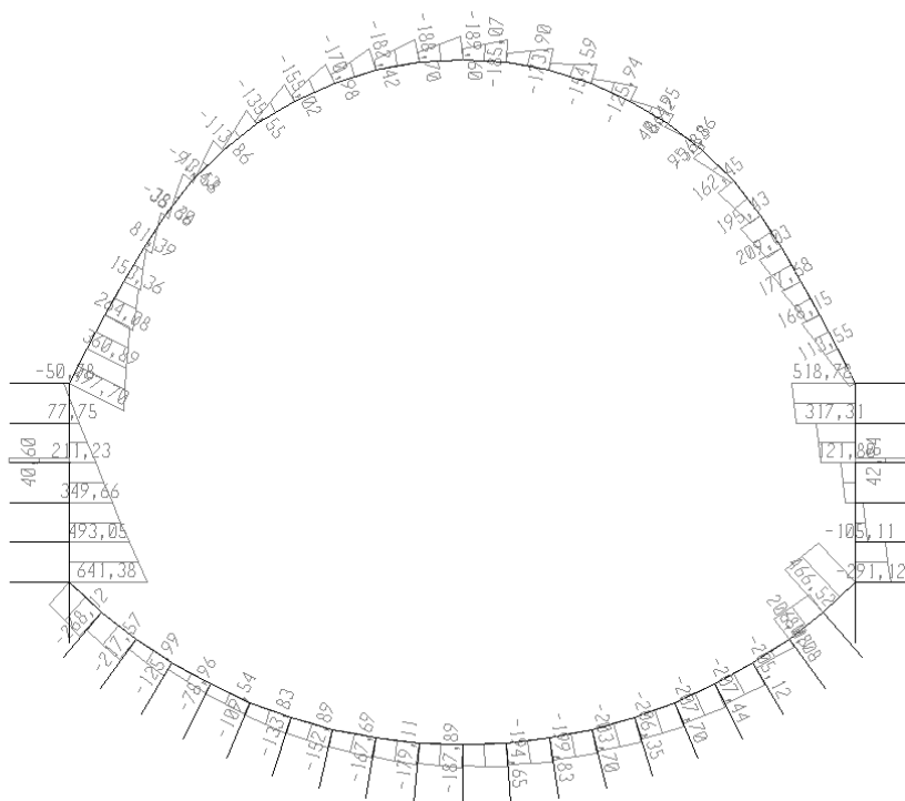
Figura 54 - COMBINAZIONE SLD- Sforzo di taglio
