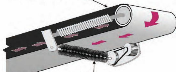
d: spazzolatore pensionato rotante in senso opposto a quello di marcia del nastro
