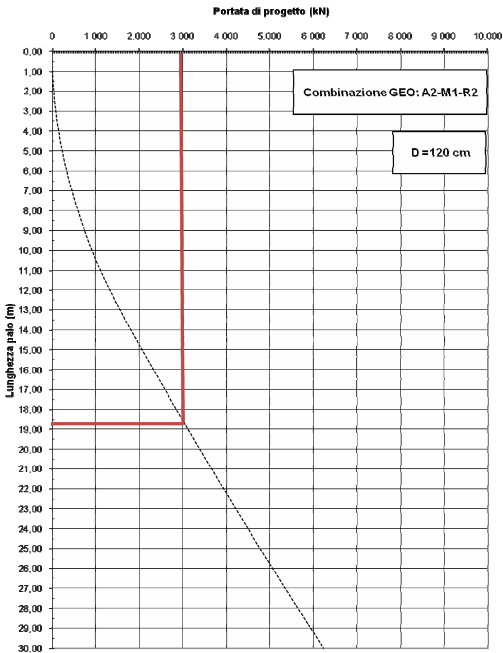
Figura 5.4: capacità portante in trazione A2-M1-R2
