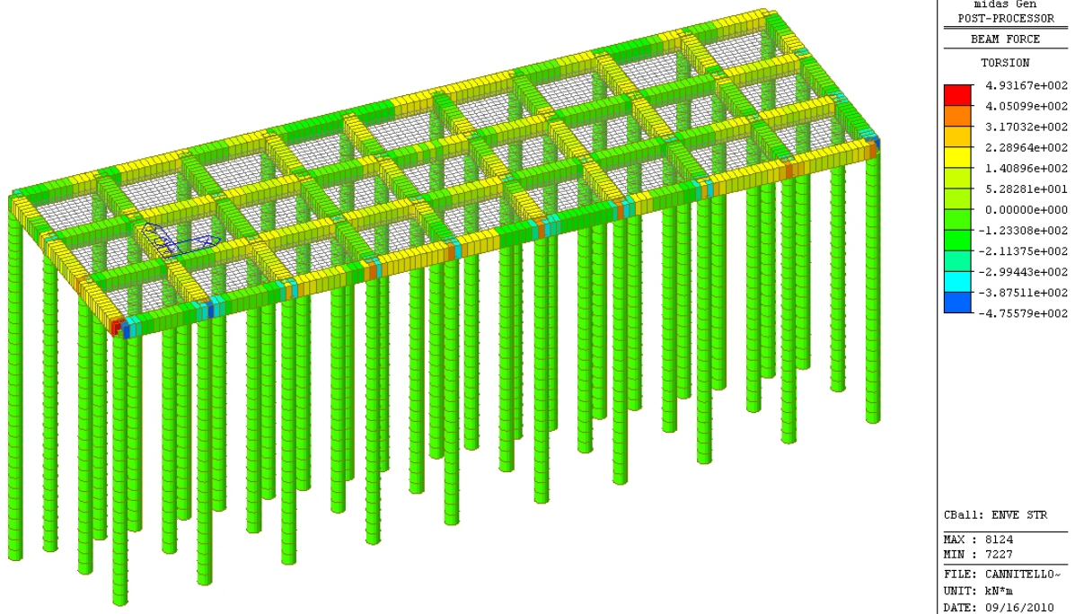
Figura 4.36: inviluppo STR: azione torcente
