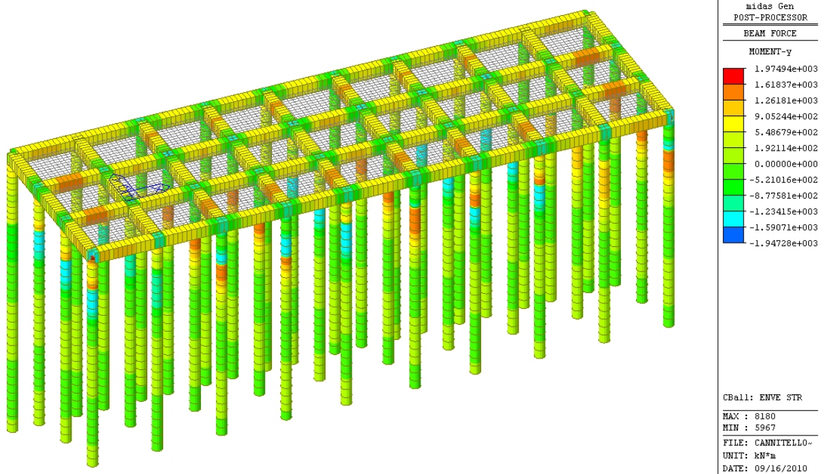
Figura 4.37: inviluppo STR: azione flettente My
