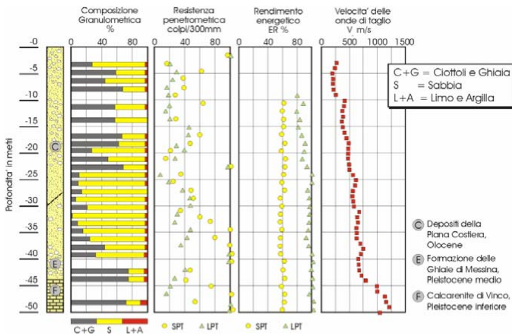
Figura 1.5: risultati prove penetrometriche SPT/LPT per la torre lato Calabria
