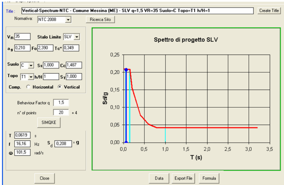
Figura 4.28: spettro di progetto verticale corrispondenza col periodo proprio in Z
