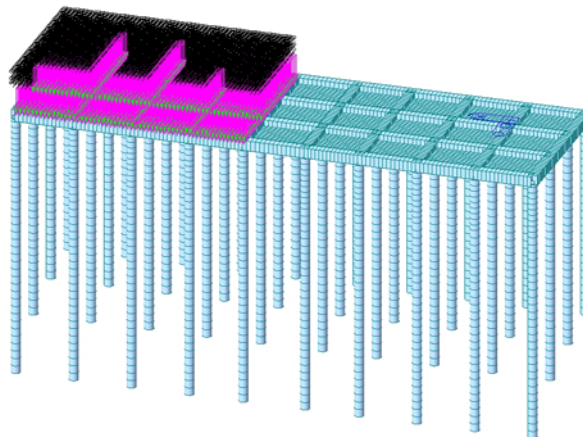
Figura 4.7: modellazione – condizione di carico: accidentali concis sx
