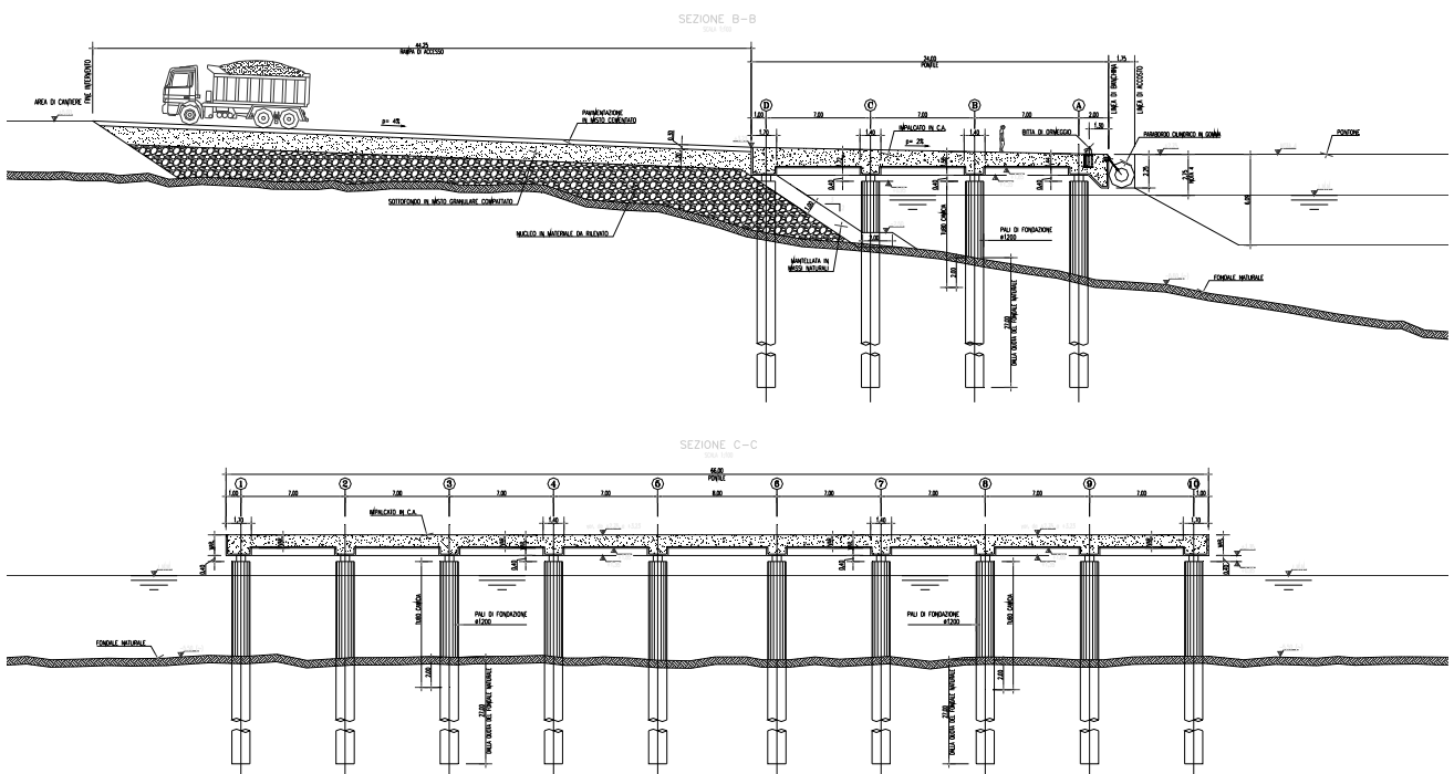
Figura 4.12: sezioni tipo dell'accosto provvisorio per l'attracco delle chiatte di trasporto conci
