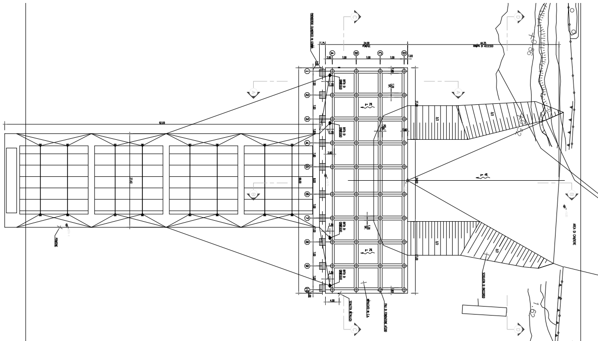
Figura 4.11: planimetria dell'accosto provvisorio per l'attracco delle chiatte di trasporto conci
