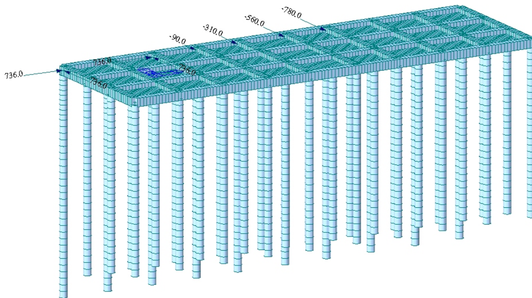
Figura 4.16: modellazione – condizione di carico:rotazione
