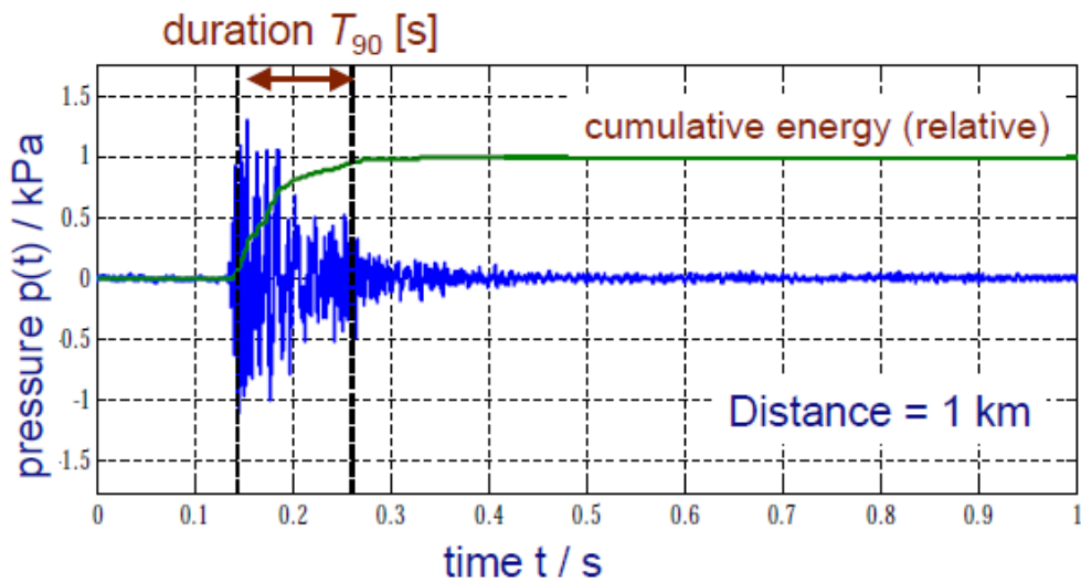
Figura 3.1 Esempio decorso temporale pressione sonora per la battitura di un palo
