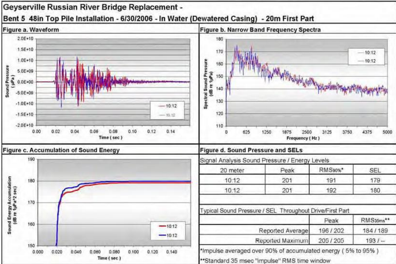
Figura 3.3 Analisi del segnale a 20 m dal palo nelle prime fasi di battitura, in assenza di acqua all'interno della camicia
