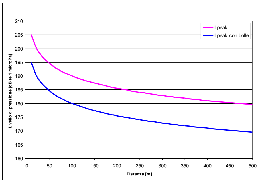
Figura 3.10 Correlazione livello di pressione sonora-distanza
