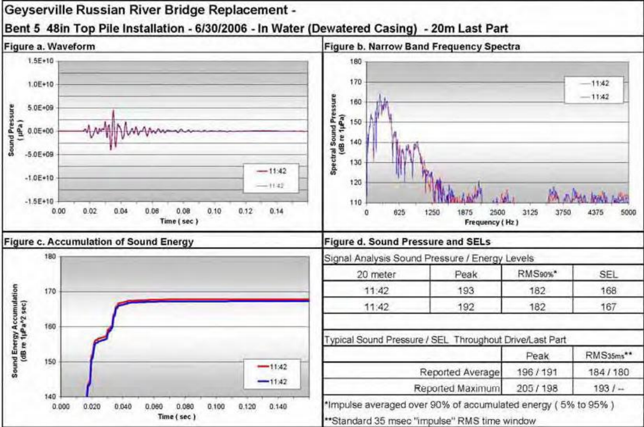
Figura 3.5 Analisi del segnale a 20 m dal palo a fine battitura, in assenza di acqua all'interno della camicia
