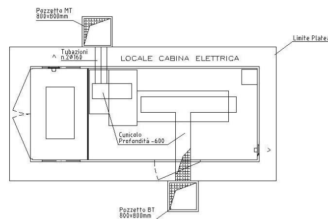
VISTA IN PIANTA Cunicoli in Platea
