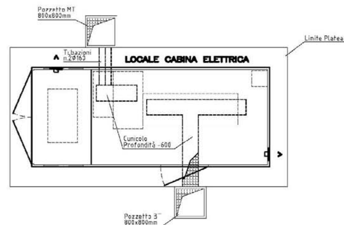
VISTA IN PIANTA Cunicoli in Platea
