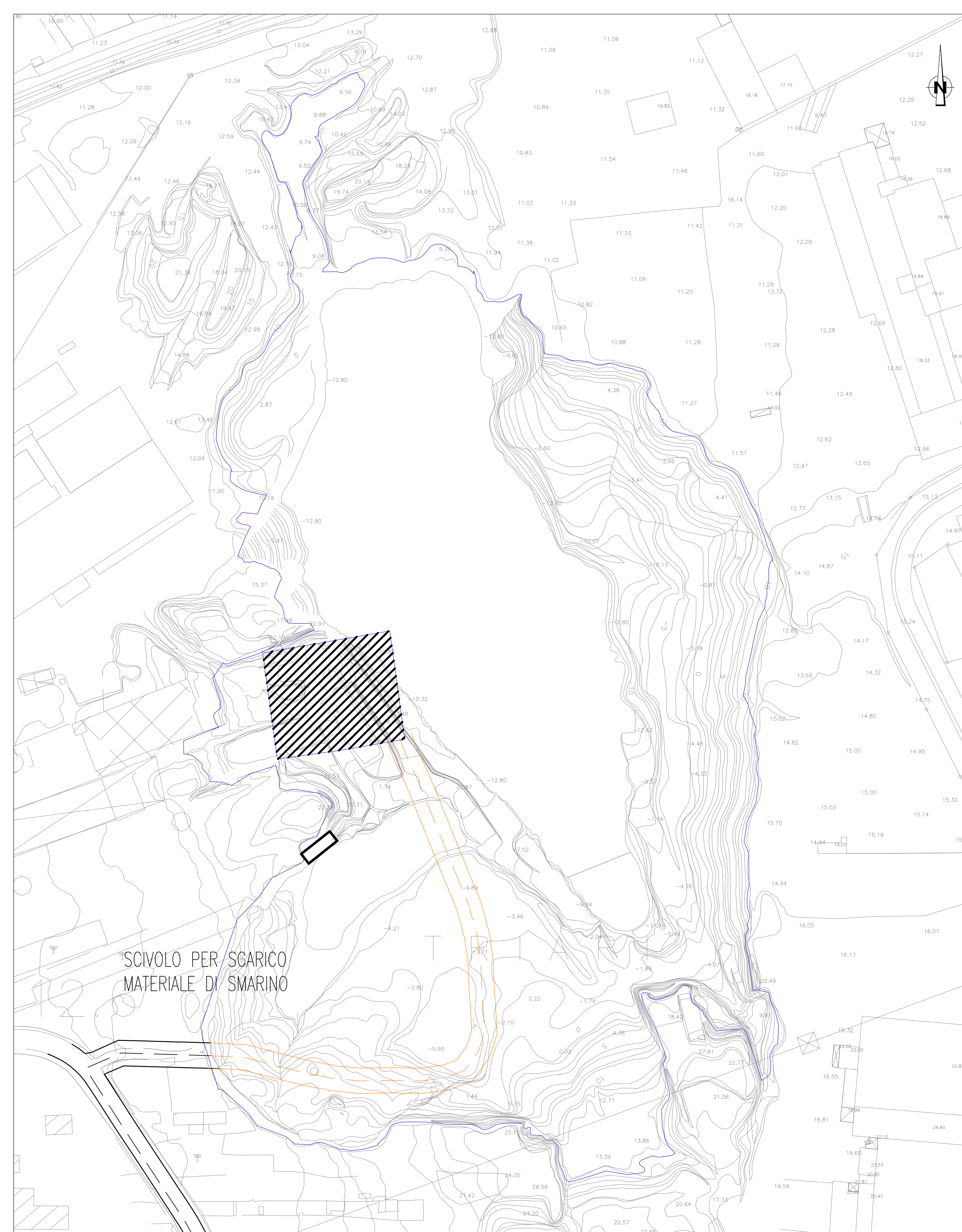
PLANIMETRIA POSIZIONAMENTO VASCA DI STOCCAGGIO TEMPORANEO E SISTEMA DI DEPURAZIONE ACQUE E VIABILITA' - FASE 2 SCALA 1:1000
