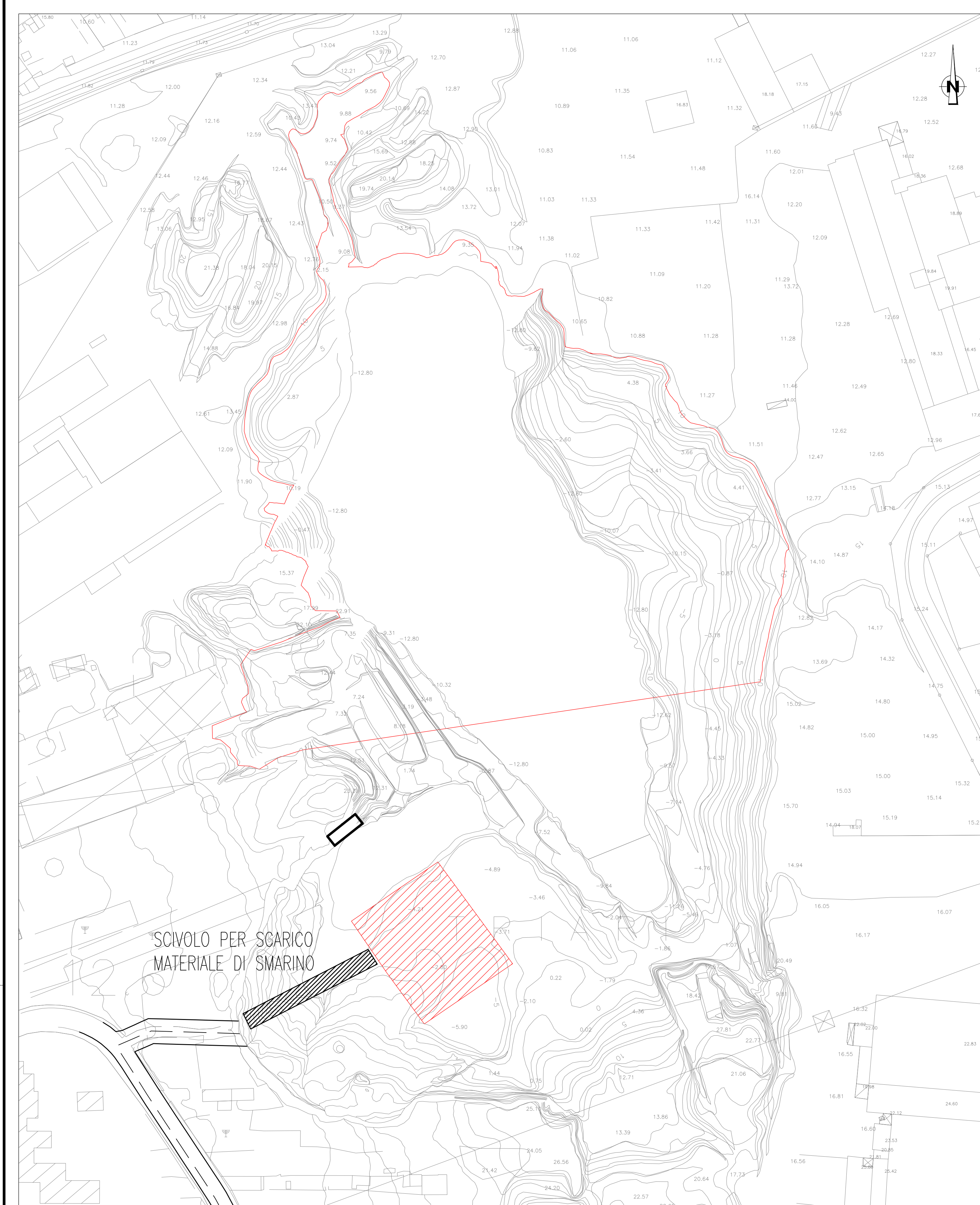
PLANIMETRIA POSIZIONAMENTO SCIVOLO, VASCA DI STOCCAGGIO TEMPORANEO E SISTEMA DI DEPURAZIONE ACQUE - FASE 1 SCALA 1:1000
