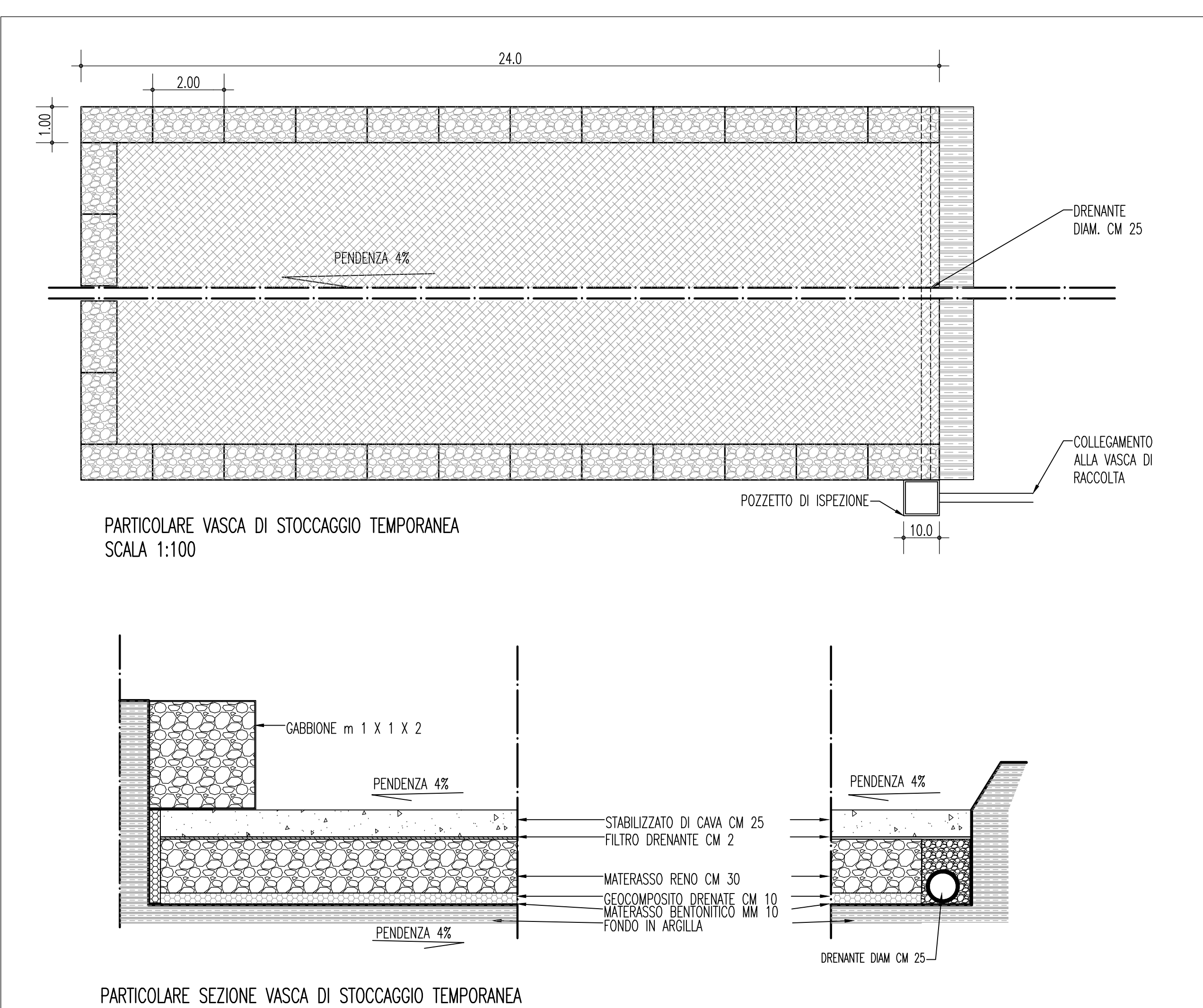
PARTICOLARE SEZIONE VASCA DI STOCCAGGIO TEMPORANEA
