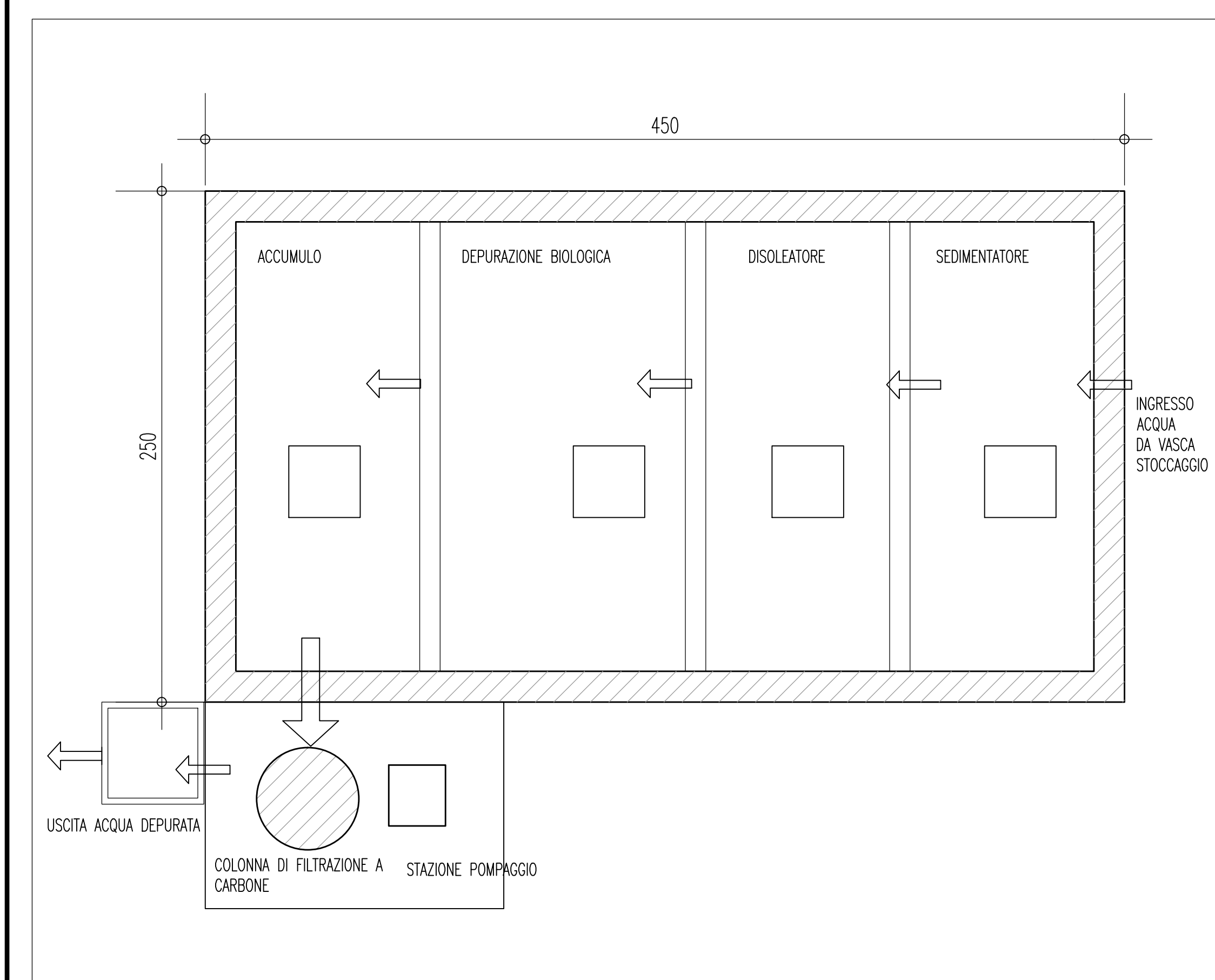
PLANIMETRIA PARTICOLARE DEPURATORE PERCOLATO VASCA DI STOCCAGGIO SCALA 1:50
