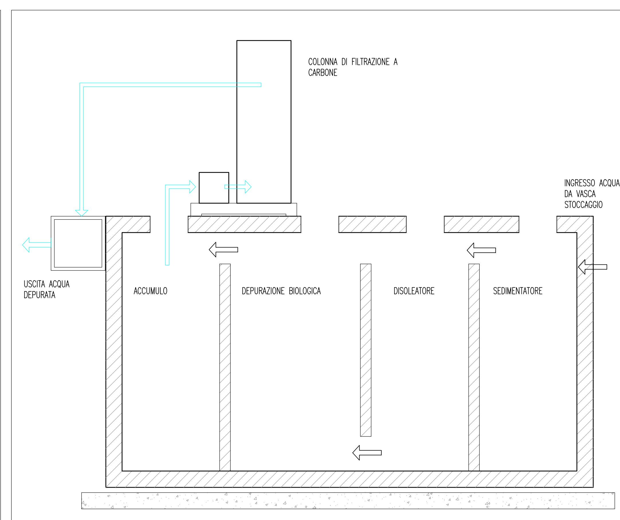
SEZIONE PARTICOLARE DEPURATORE PERCOLATO VASCA DI STOCCAGGIO SCALA 1:50
