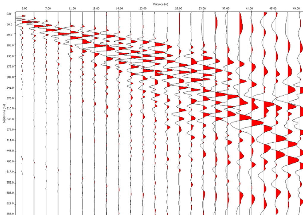
Figura 3.1: Tracce sperimentali
