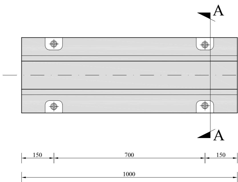
PIANTA
