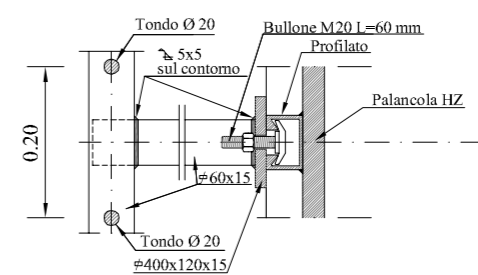
DETTAGLIO "B" SCALA 1:10 SEZIONE
