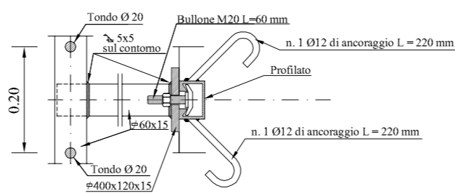
DETTAGLIO "A" SCALA 1:10 SEZIONE
