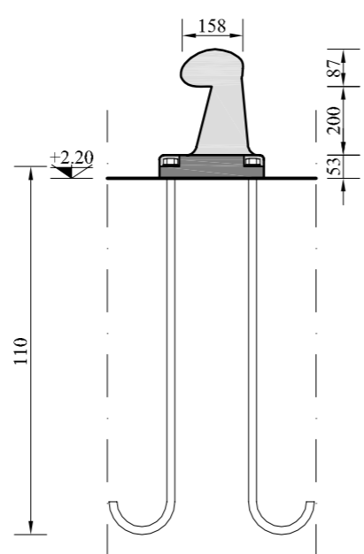
VISTA LATERALE
