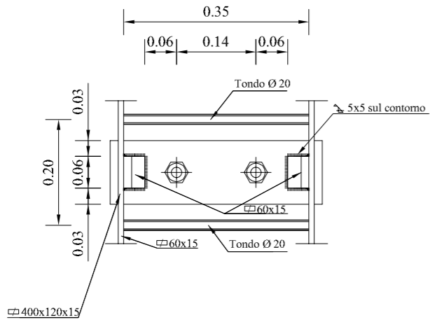
VISTA DETTAGLI "A" E "B" SCALA 1:10
