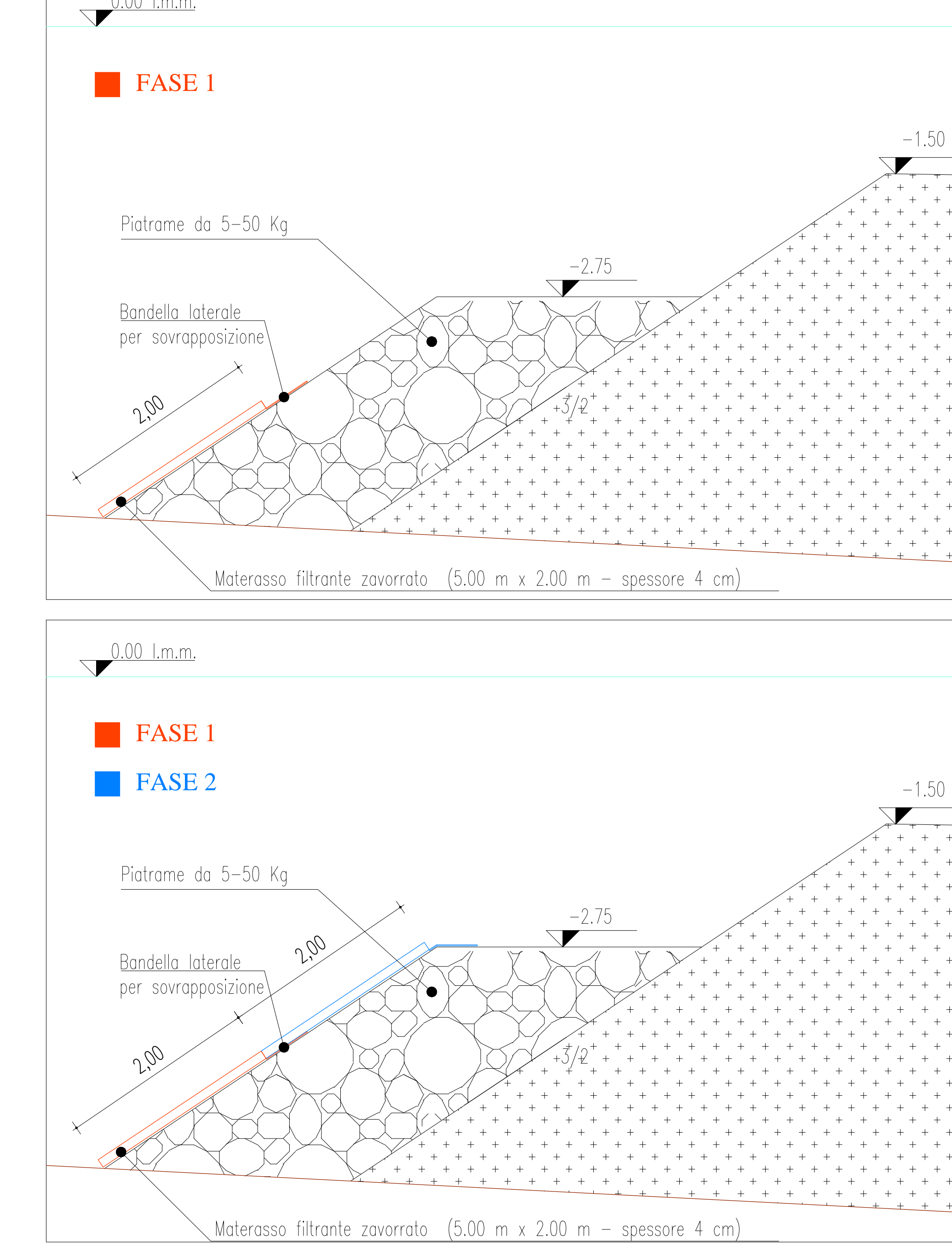
FASI DI COLLOCAZIONE MATERASSO FILTRANTE SEZIONI SCOGLIERA SOFFOLTA - SCALA 1:200
