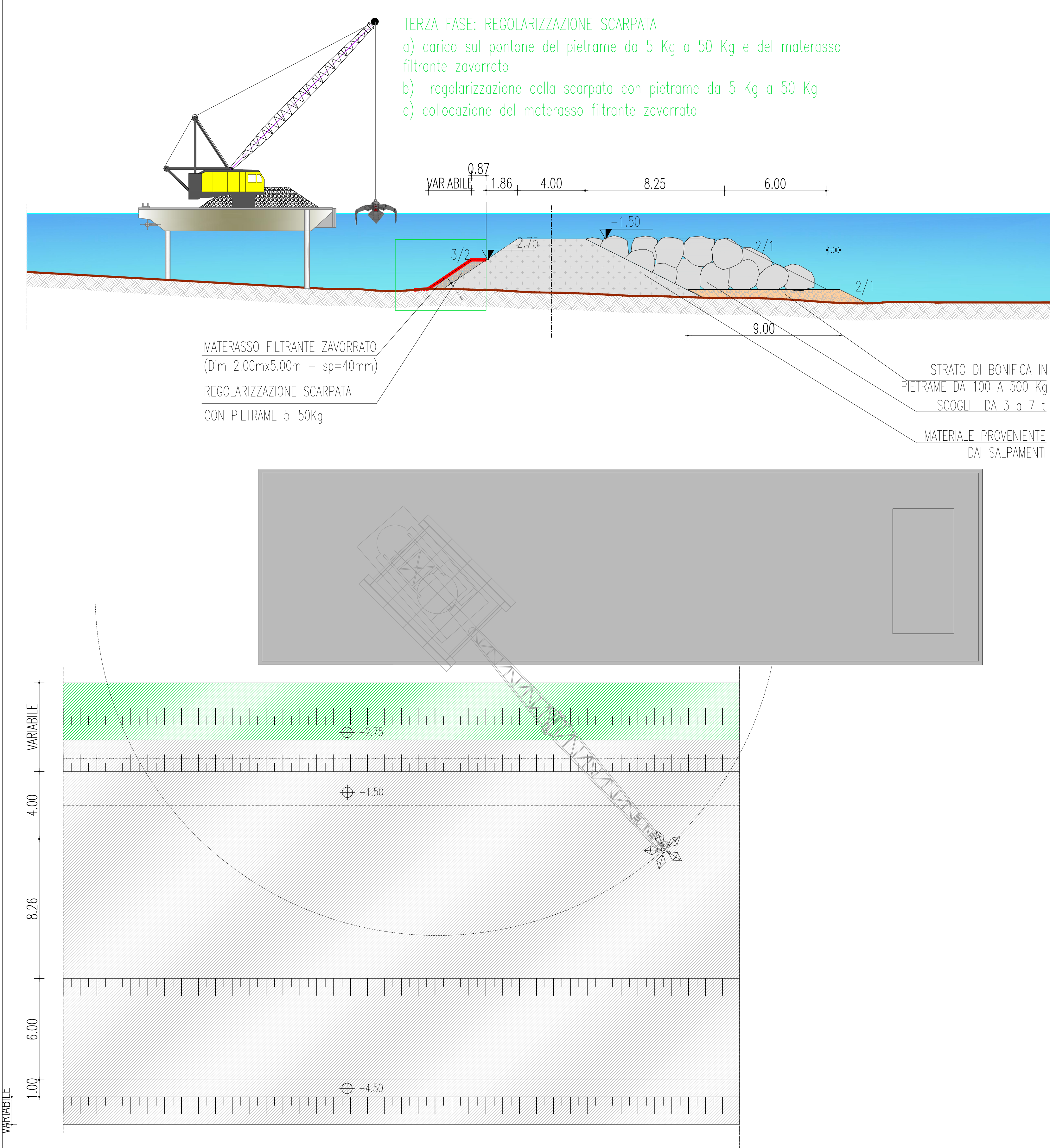
FASI DI COLLOCAZIONE MATERASSO FILTRANTE VISTA PLANIMETRICA - SCALA 1:100
