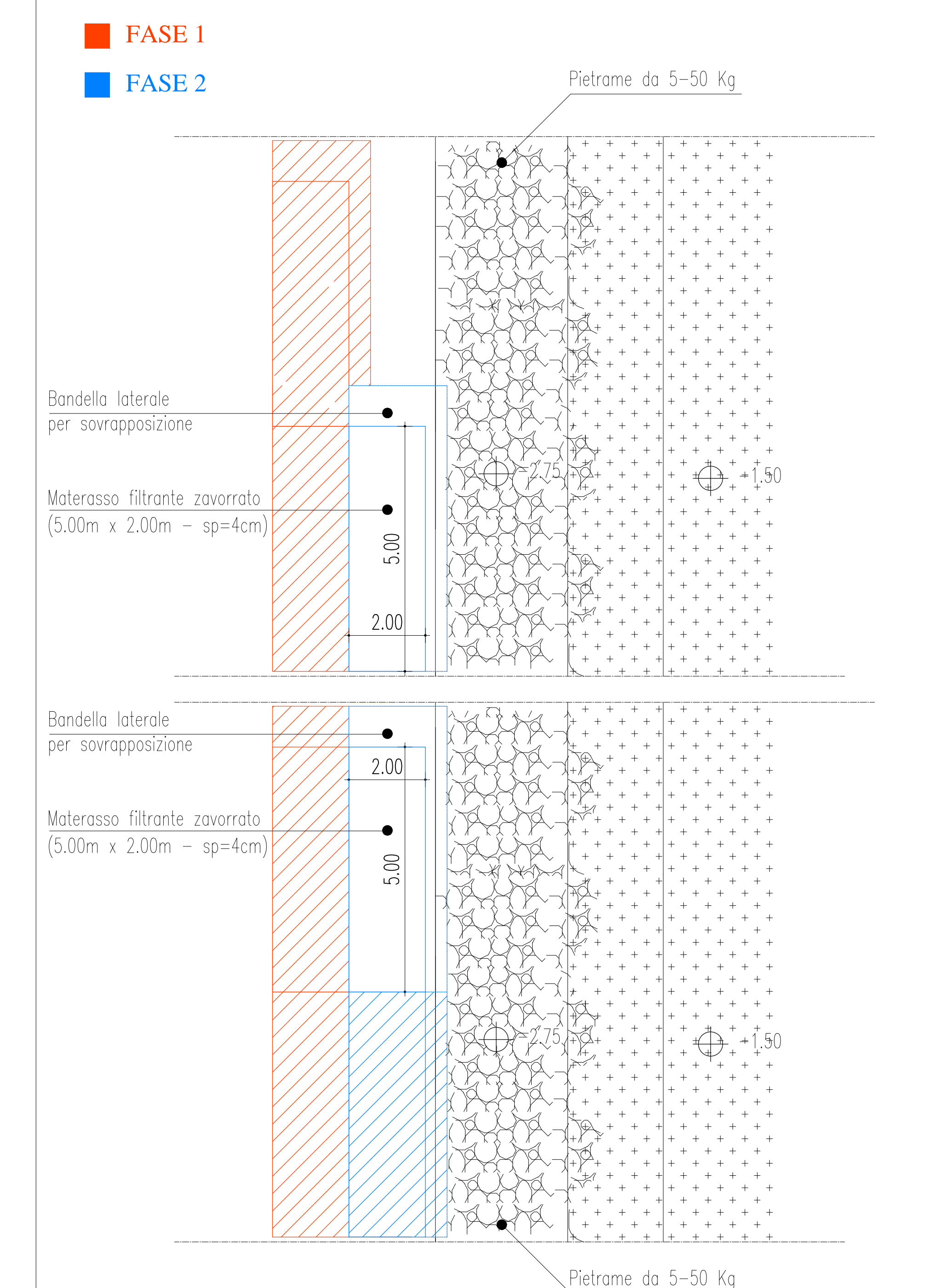
FASI DI COLLOCAZIONE MATERASSO FILTRANTE VISTA PLANIMETRICA - SCALA 1:100
