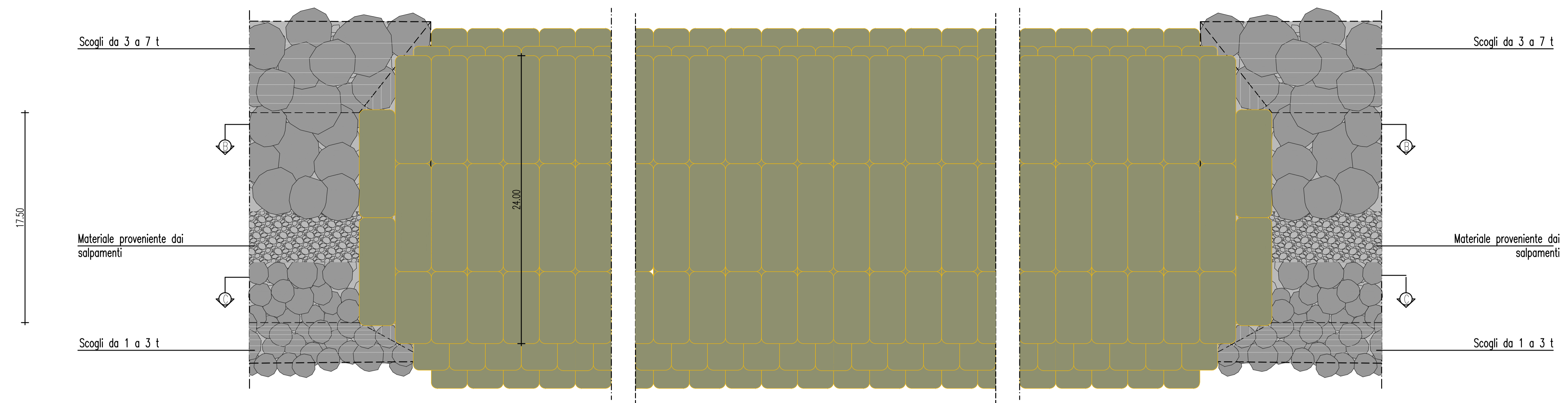
PARTICOLARE COLLEGAMENTO TIPO SCOGLIERE Scala 1:200
