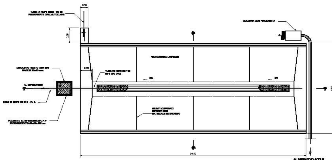
PIANTA Scala 1: 50
