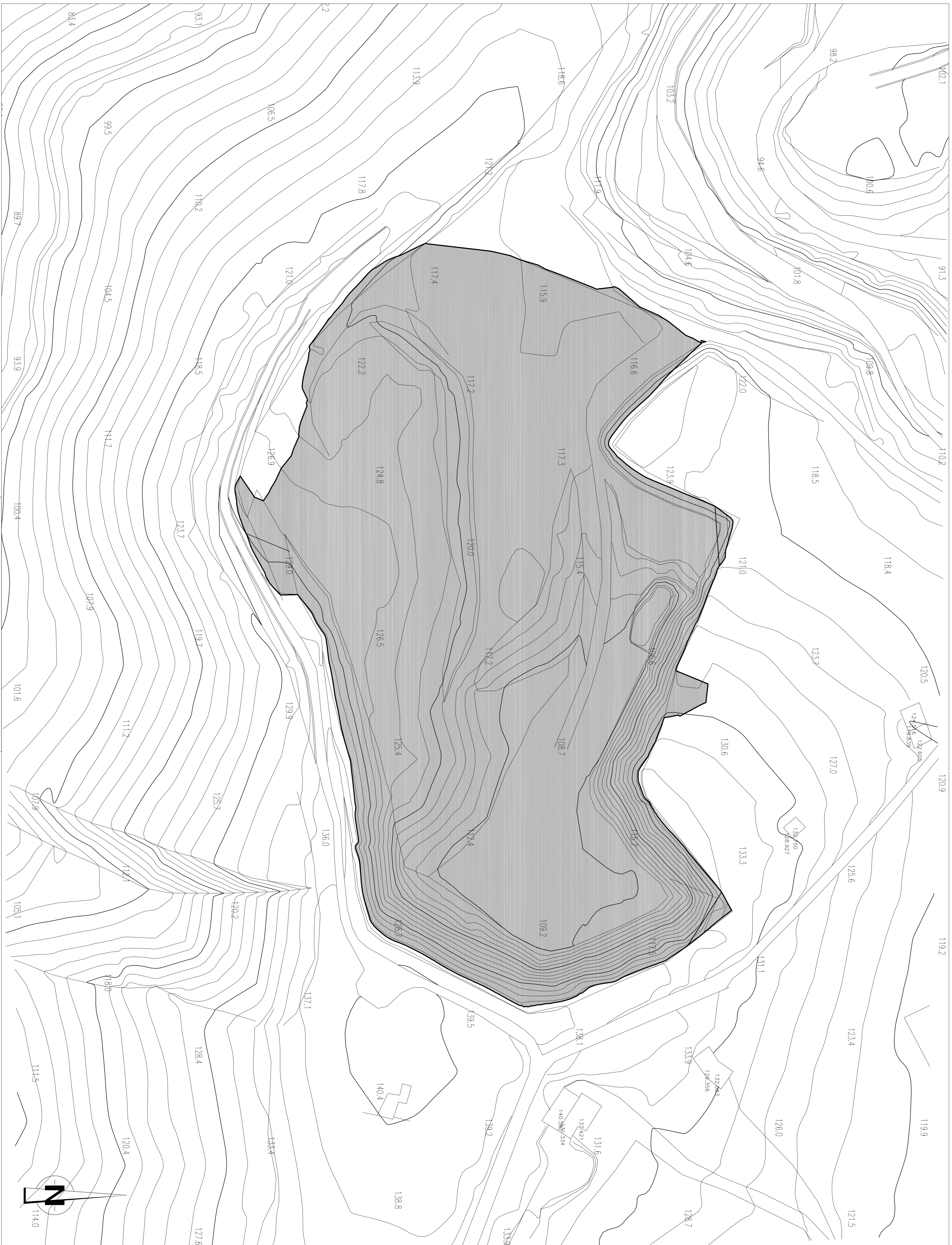
PLANIMETRIA DELLO STATO DI FATTO Scala 1:500
